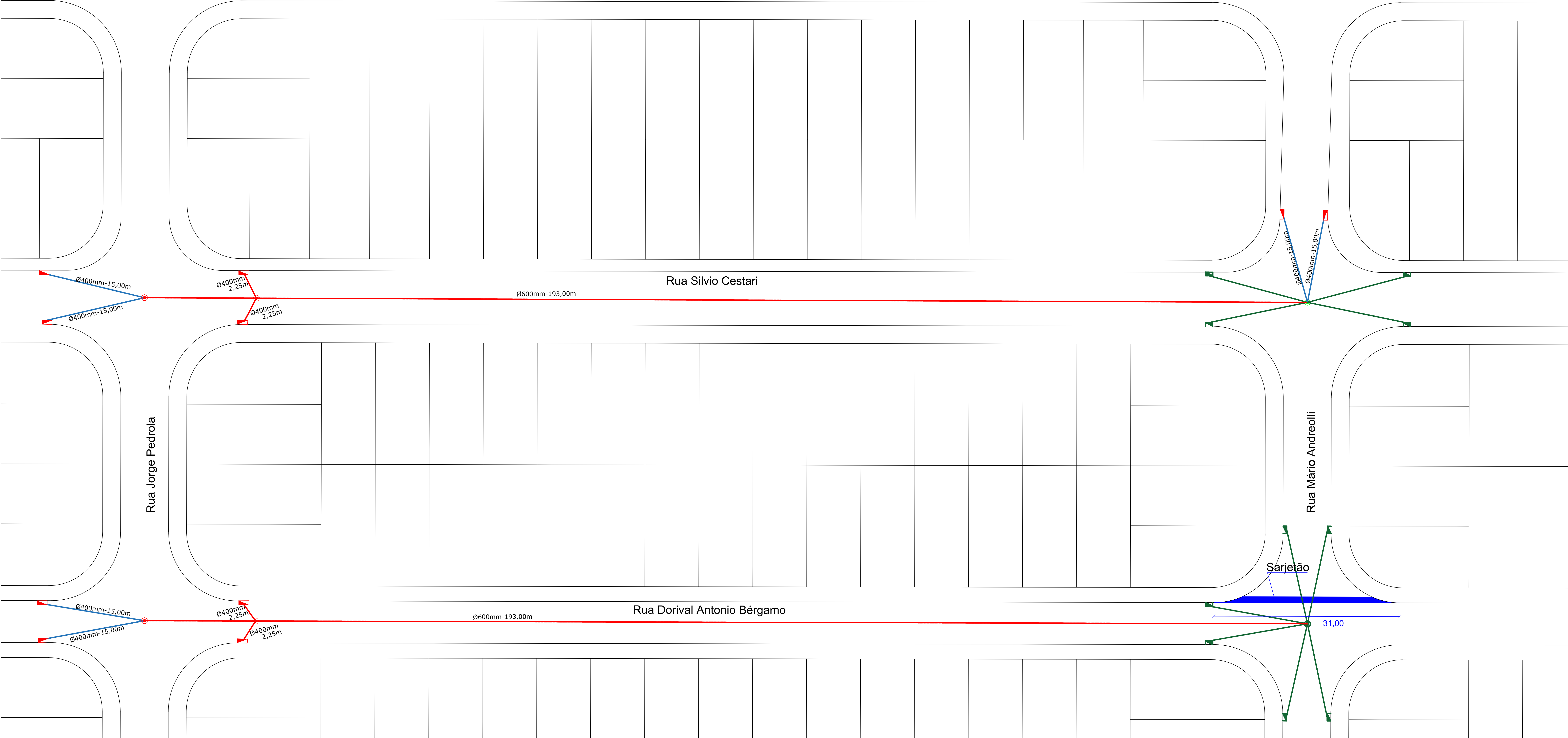
IMPLANTAÇÃO DRENAGEM PLUVIAL ESCALA 1:250
