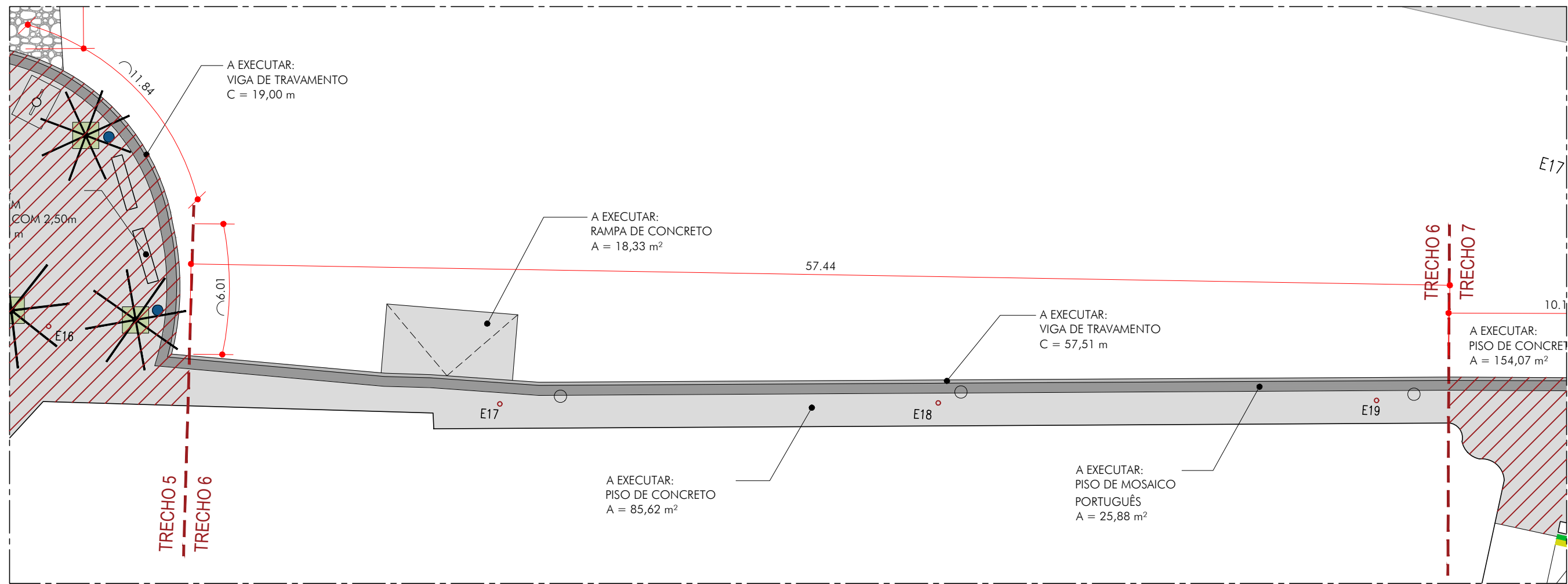
PROPOSTA - TRECHO 6 ESC. 1:200
