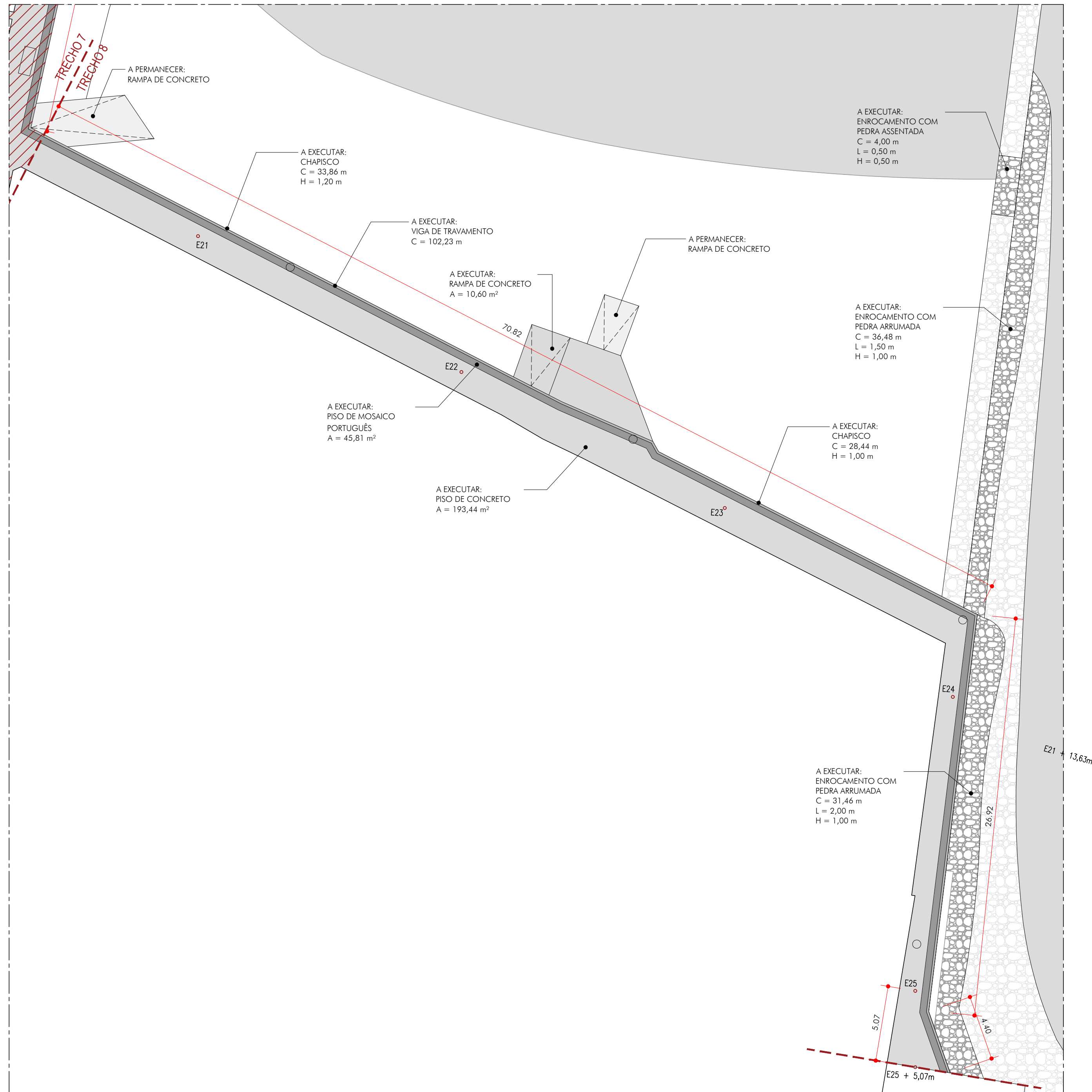
PROPOSTA - TRECHO 8 ESC. 1:200
