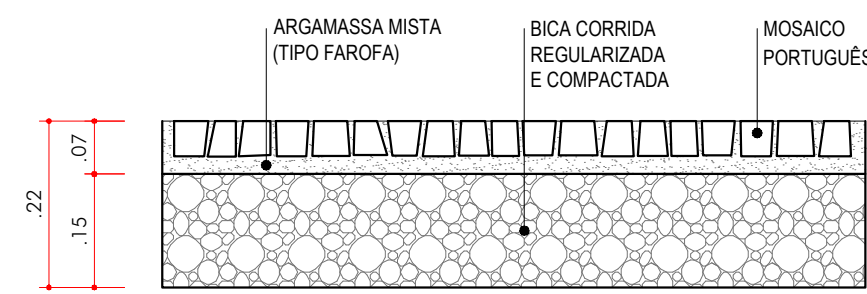
DET 02 - PISO SOBRE DEMOLIÇÃO DE PISO EXISTENTE ESC. 1:10
