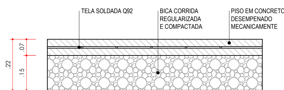
DET 01 - PISO SOBRE DEMOLIÇÃO DE PISO EXISTENTE ESC. 1:10
