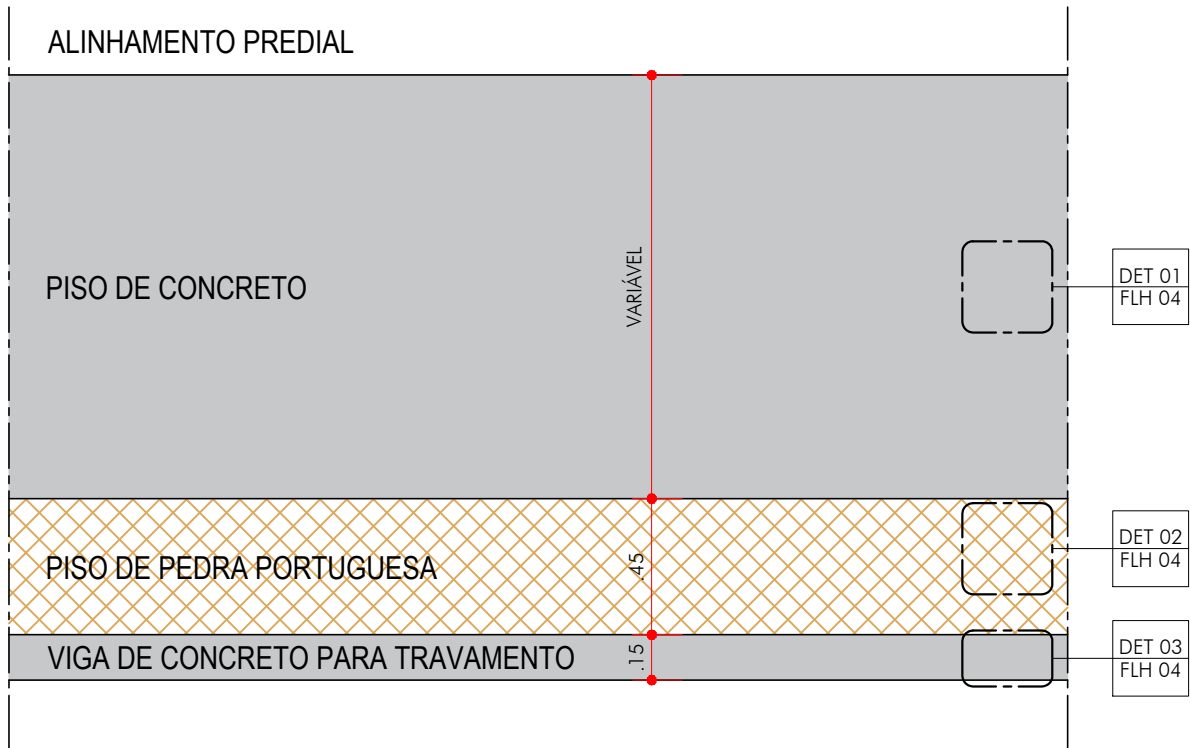
DET 01 ESC. 1:25
