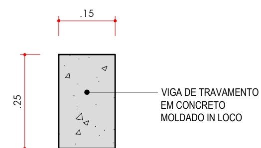
DET 03 - VIGA DE TRAVAMENTO ESC. 1:10
