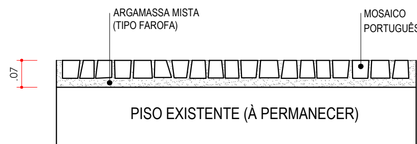
DET 02- PISO SOBRE PISO EXISTENTE ESC. 1:10
