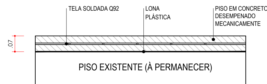
DET 01 - PISO SOBRE PISO EXISTENTE ESC. 1:10
