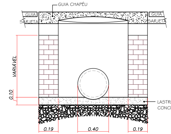
DETALHE 2
