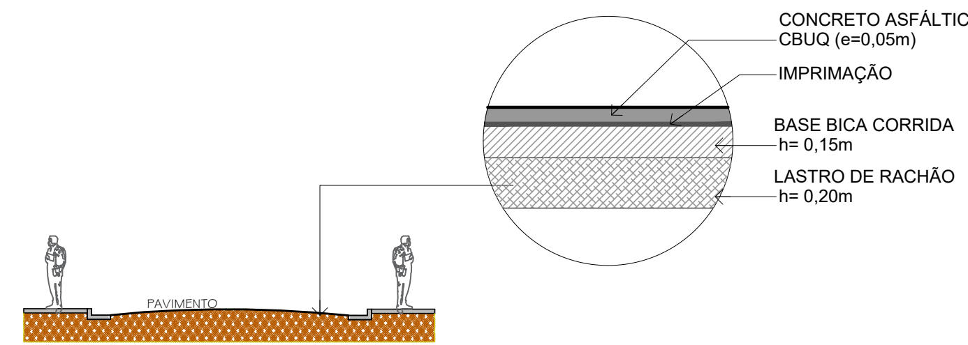
SEÇÃO TÍPICA DO PAVIMENTO CORTE ESQUEMÁTICO BB ESCALA 1:125
