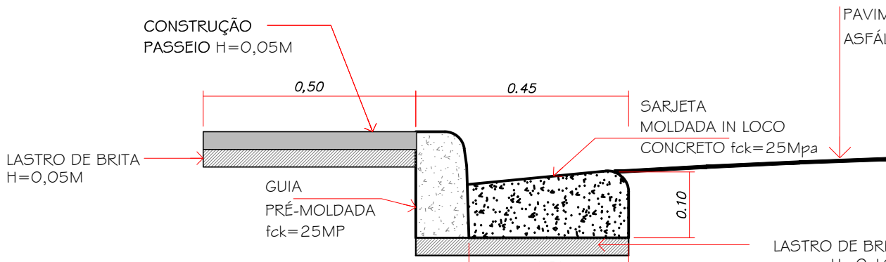
DETALHE - GUIA/SARJETA GERAL ESCALA 1:15
