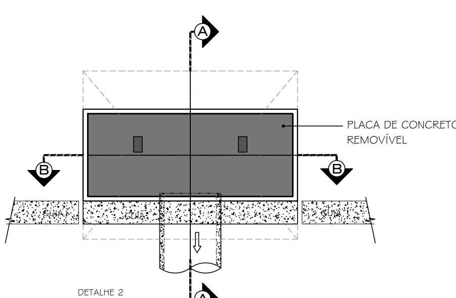
DETALHE 2 BOCA DE LOBO
