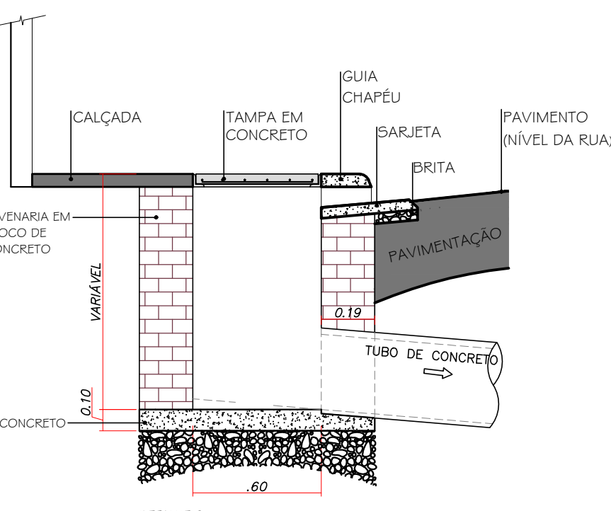
DETALHE 2 CORTE AA
