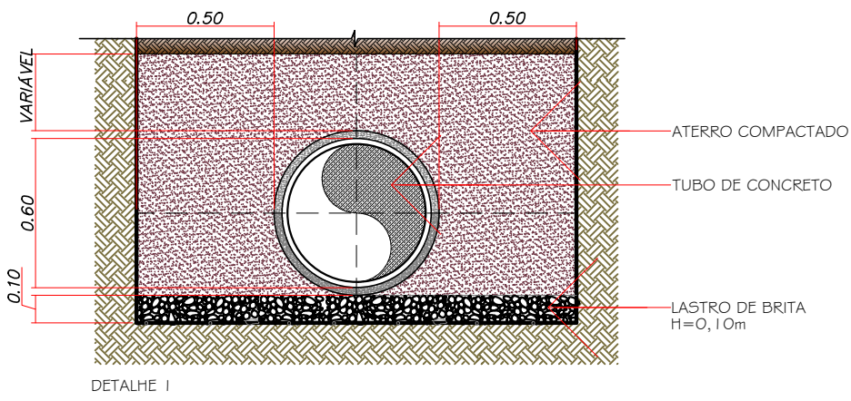
DETALHE 1
