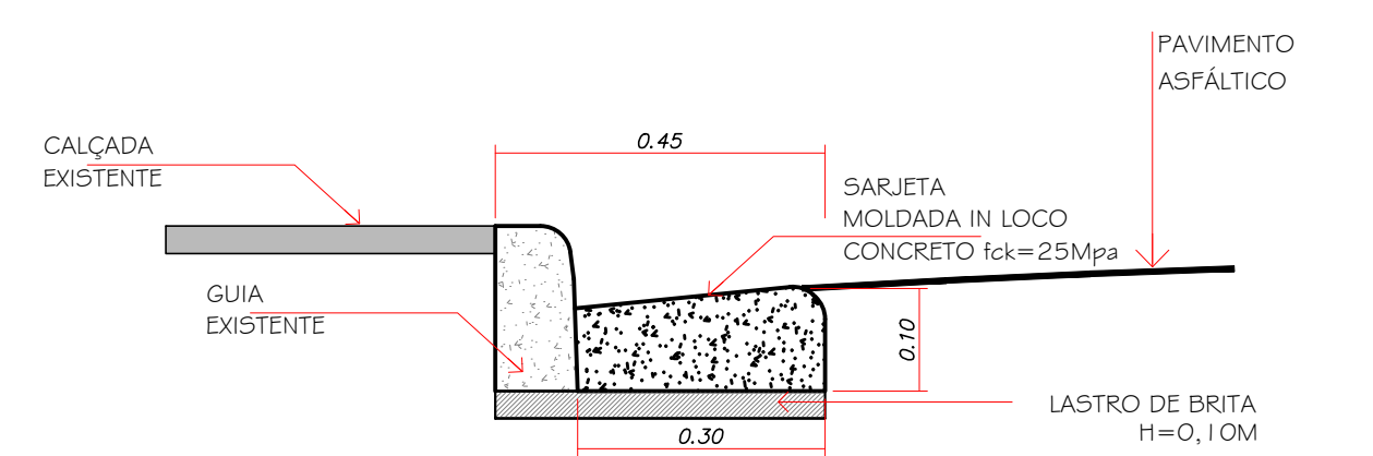
DETALHE - SARJETA GERAL ESCALA 1:15
