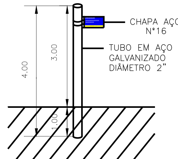
DETALHE PLACAS DE LOGRADOURO ESCALA 1:50
