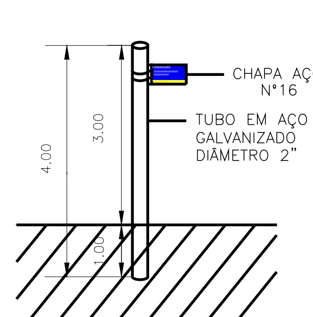
DETALHE PLACAS DE LOGRADOURO ESCALA 1:50
