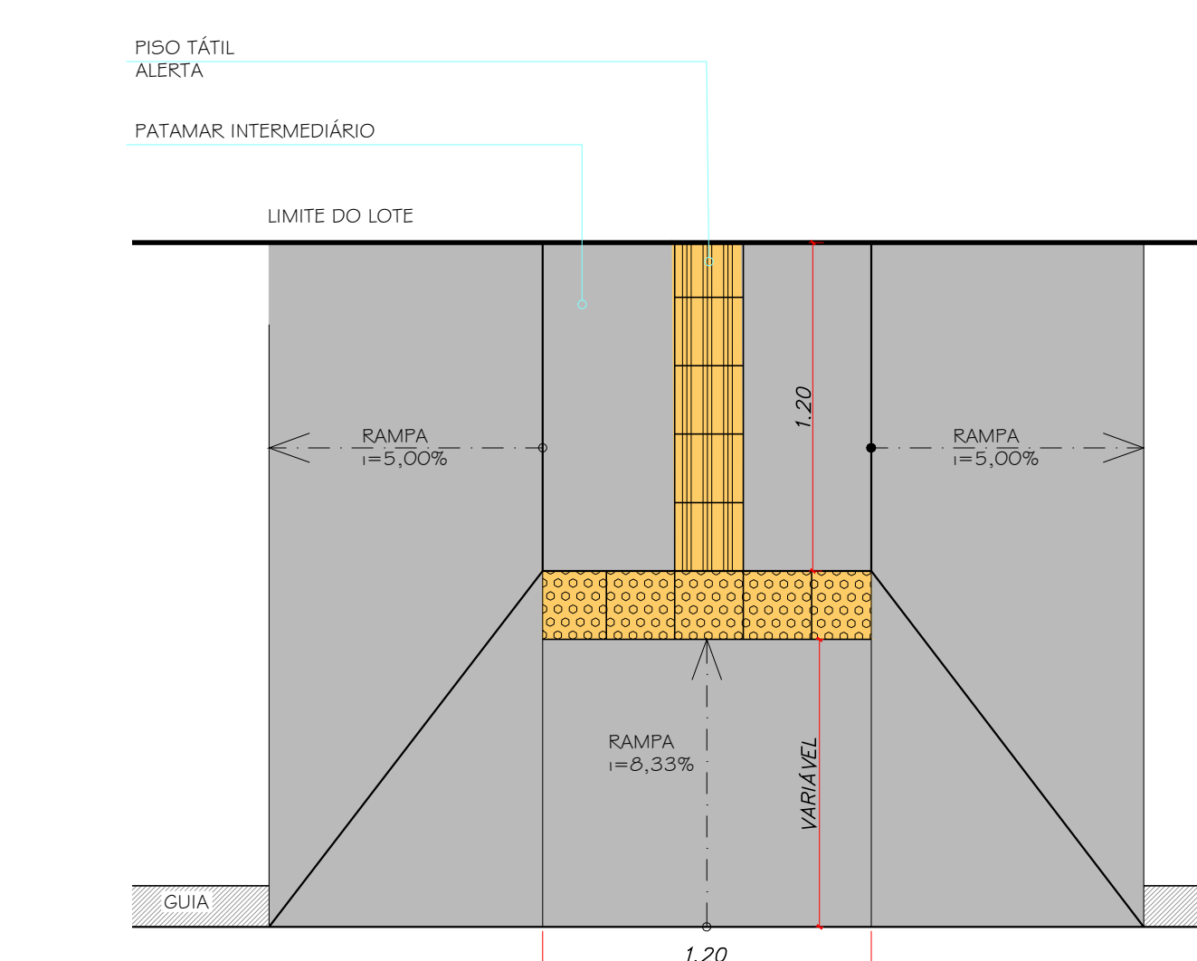
DETALHE RAMPA ACESSIBILIDADE - TIPO 1 ESCALA 1:25
