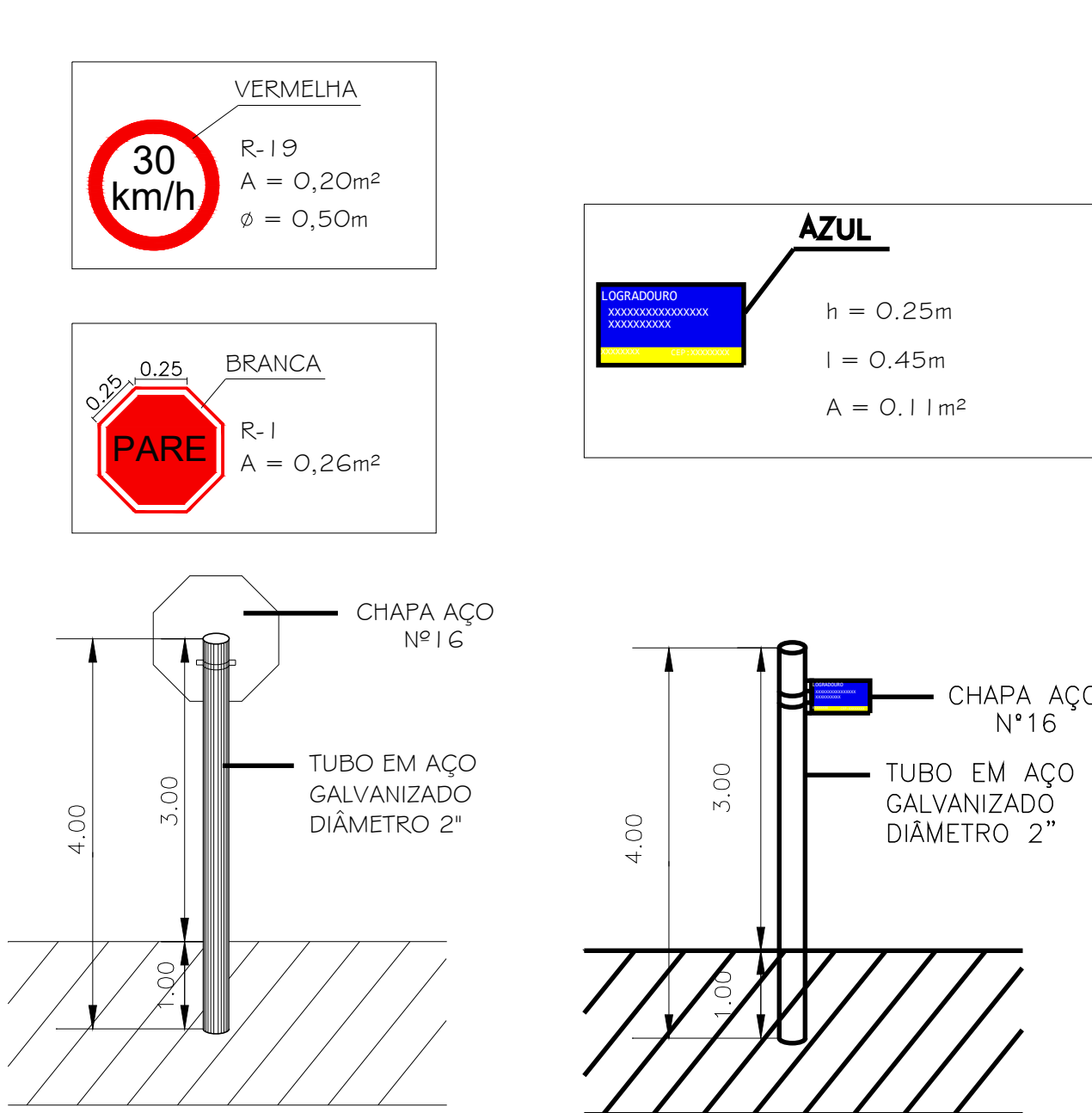
DETALHE PLACAS DE SINALIZAÇÃO VERTICAL ESCALA 1:50
