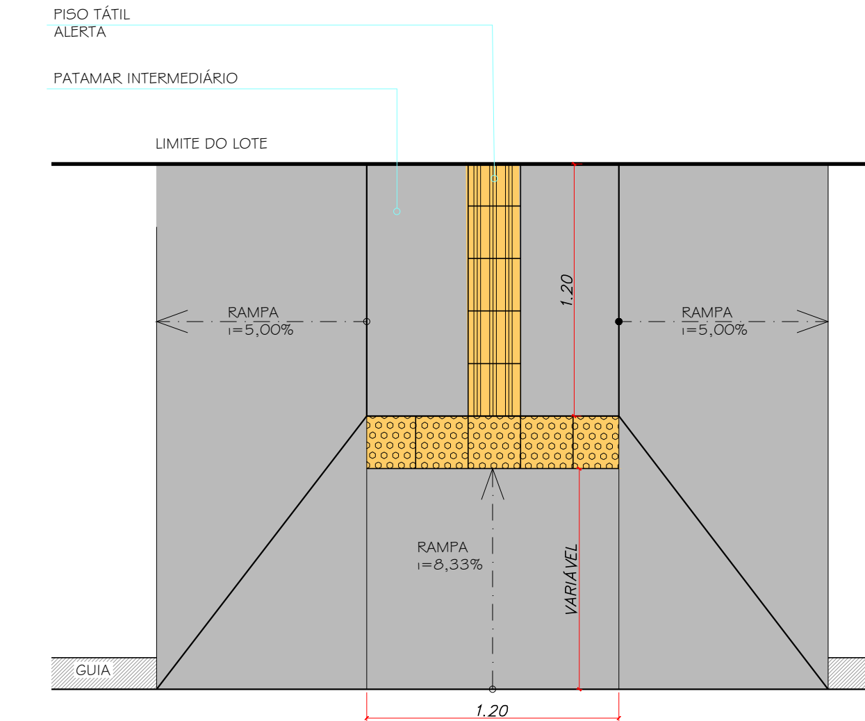
DETALHE RAMPA ACESSIBILIDADE - TIPO 1 ESCALA 1:25
