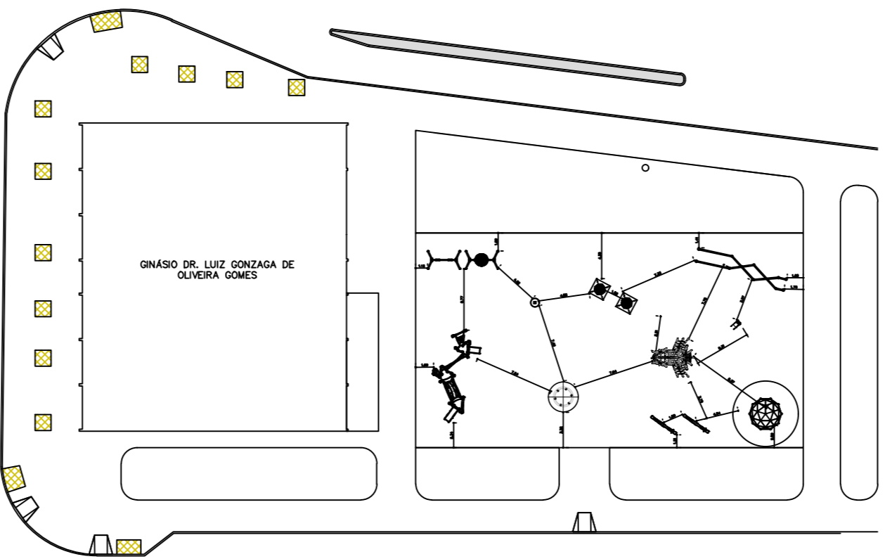
PLAYGROUND – PLANTA MEDIDAS DE POSICIONAMENTO BRINQUEDOS ESC. 1:100
