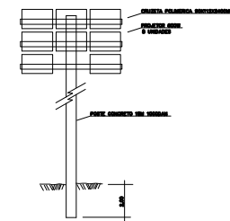
DET. POSTE PROJETORES
