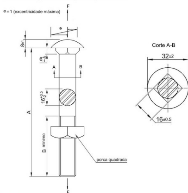
Figura 2: Detalhes Parafuso 16x70mm
