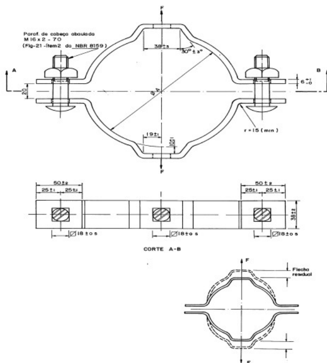
Figura 1: Detalhes Cinta de Aço
