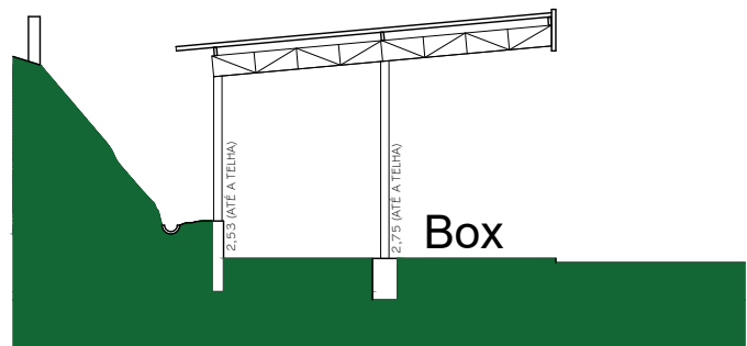
CORTE C-C
