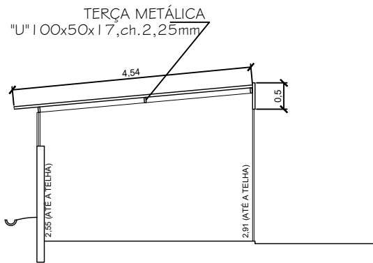
CORTE B-B
