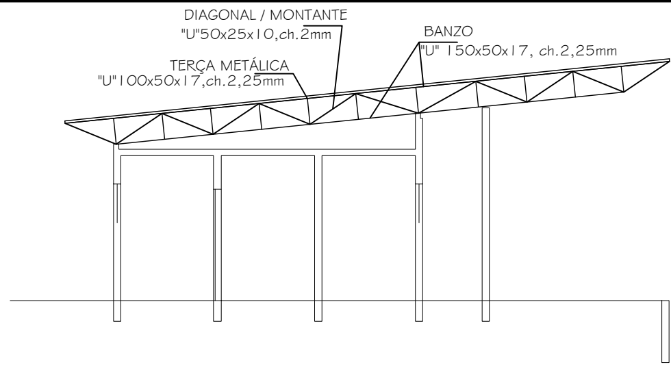
CORTE A-A
