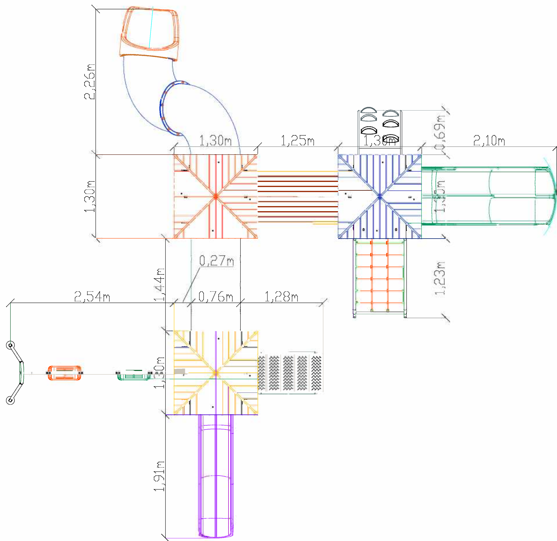
① PLANTA BAIXA PLAYGROUND ESC. 1:25
