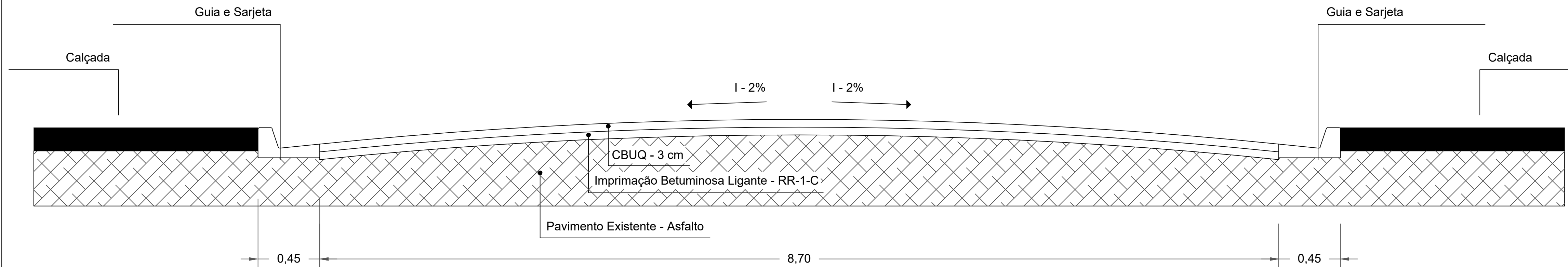
PERFIL DAS VIAS SEM ESCALA
