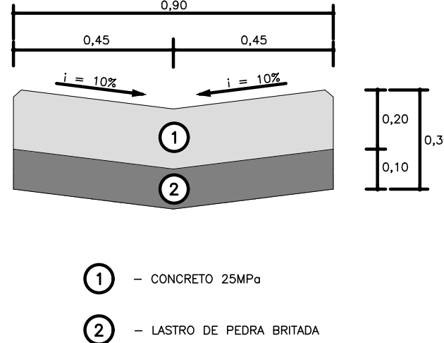
SARJETÃO EM CONCRETO L=0,90m SEM ESCALA
