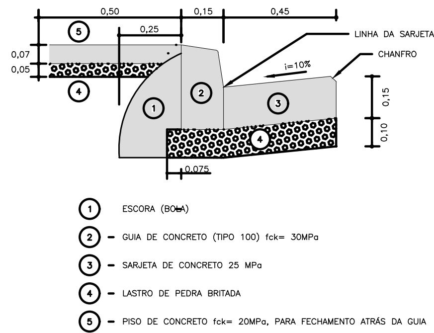
DETALHE DE GUIA E SARJETA 0,45m SEM ESCALA
