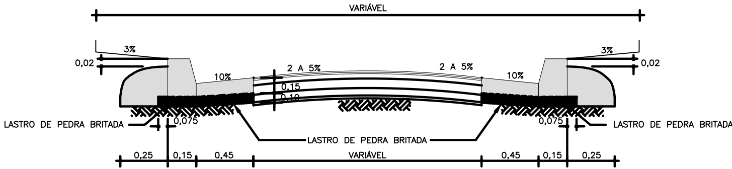
SEÇÃO TÍPICA PAVIMENTAÇÃO ASFÁLTICA SEM ESCALA
