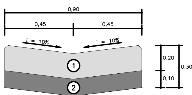
SARJETÃO EM CONCRETO L=0,90m
