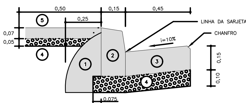
DETALHE DE GUIA E SARJETA 0,45m
