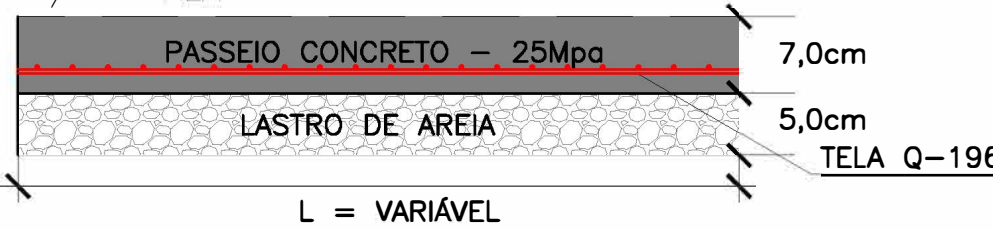
DETALHE - SEÇÃO DE CALÇAMENTO S/ ESCALA
