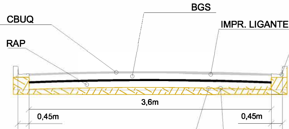
SEÇÃO-TIPO DE PAVIMENTAÇÃO 8/ ESC.
