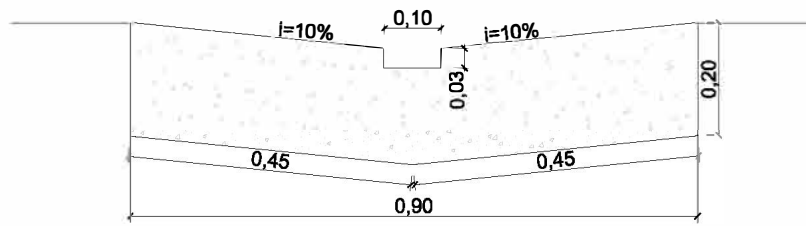
DETALHE DE SARJETÃO ESCALA 1:20
