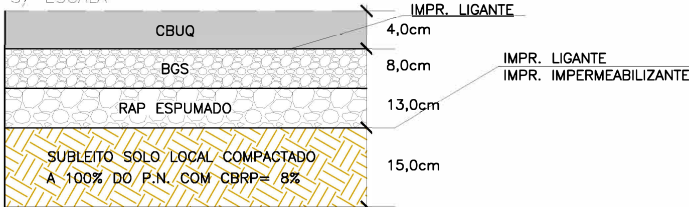
DETALHE TÍPICO - SEÇÃO DE PAVIMENTO S/ ESCALA
