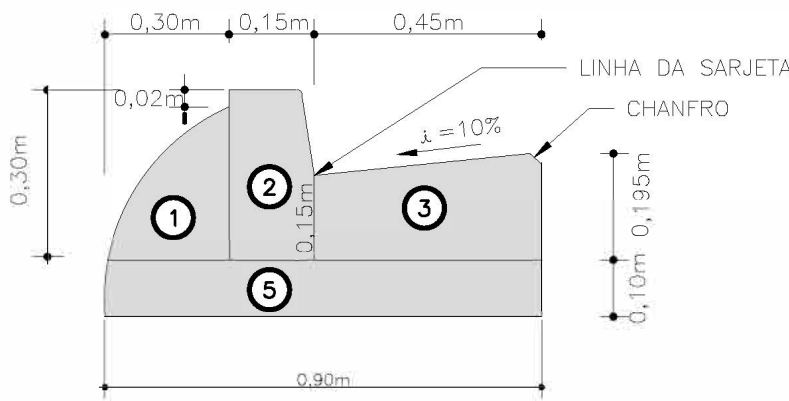
DETALHE TÍPICO DE GUIA E SARJETA 0,45m SEM ESCALA
