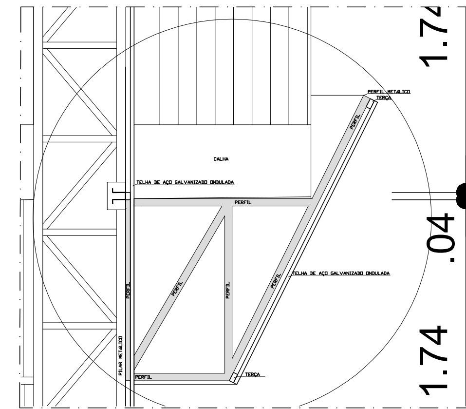
7 DETALHE 01 - PERFIL METÁLICO 1 ESC 1:20
