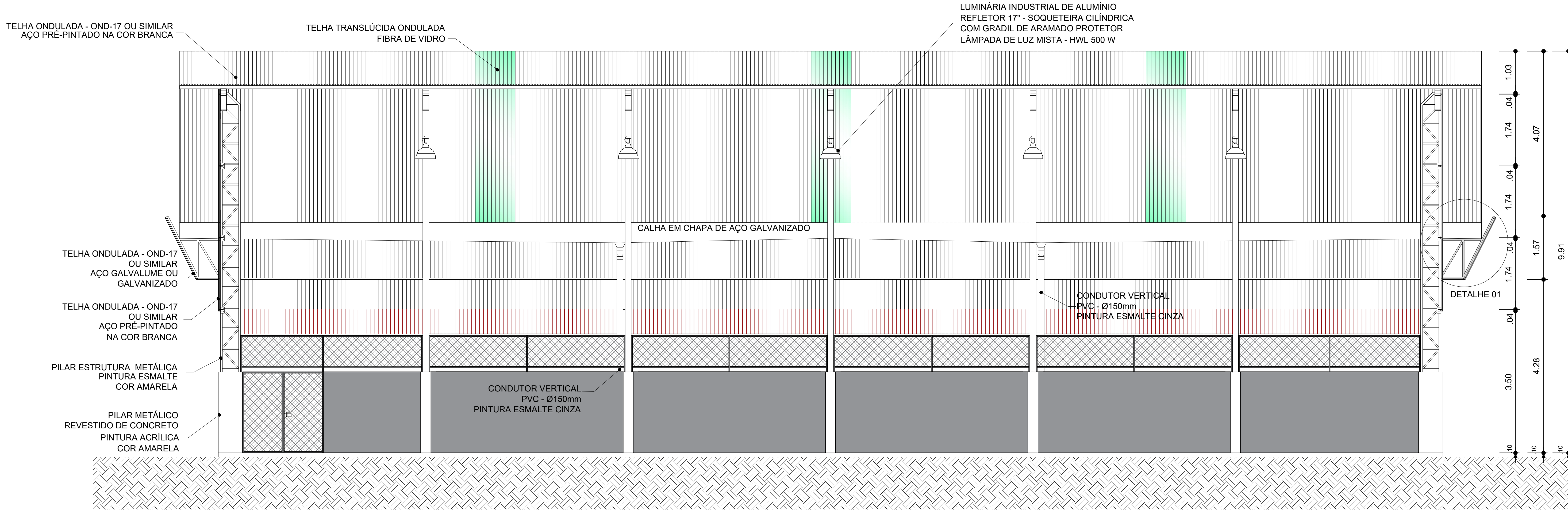
5 CORTE AA 1:50
