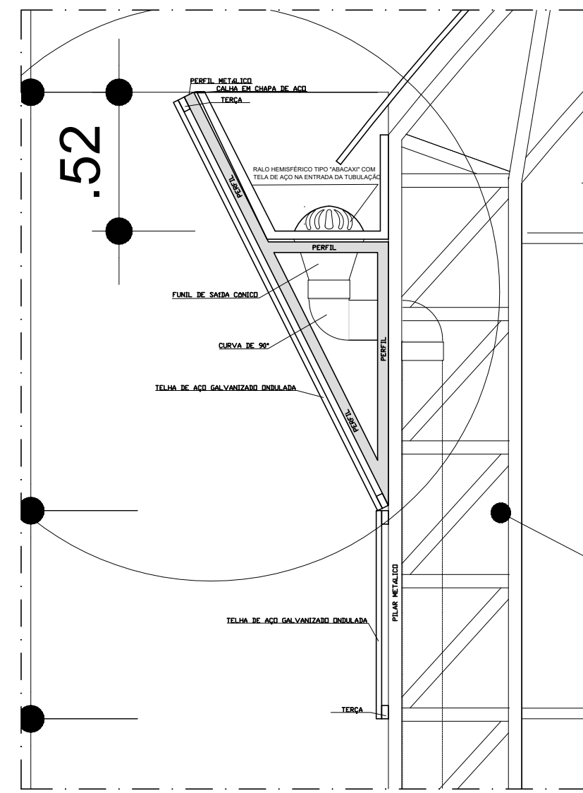
8 DETALHE 02 - PERFIL METÁLICO 2 ESC 1:20
