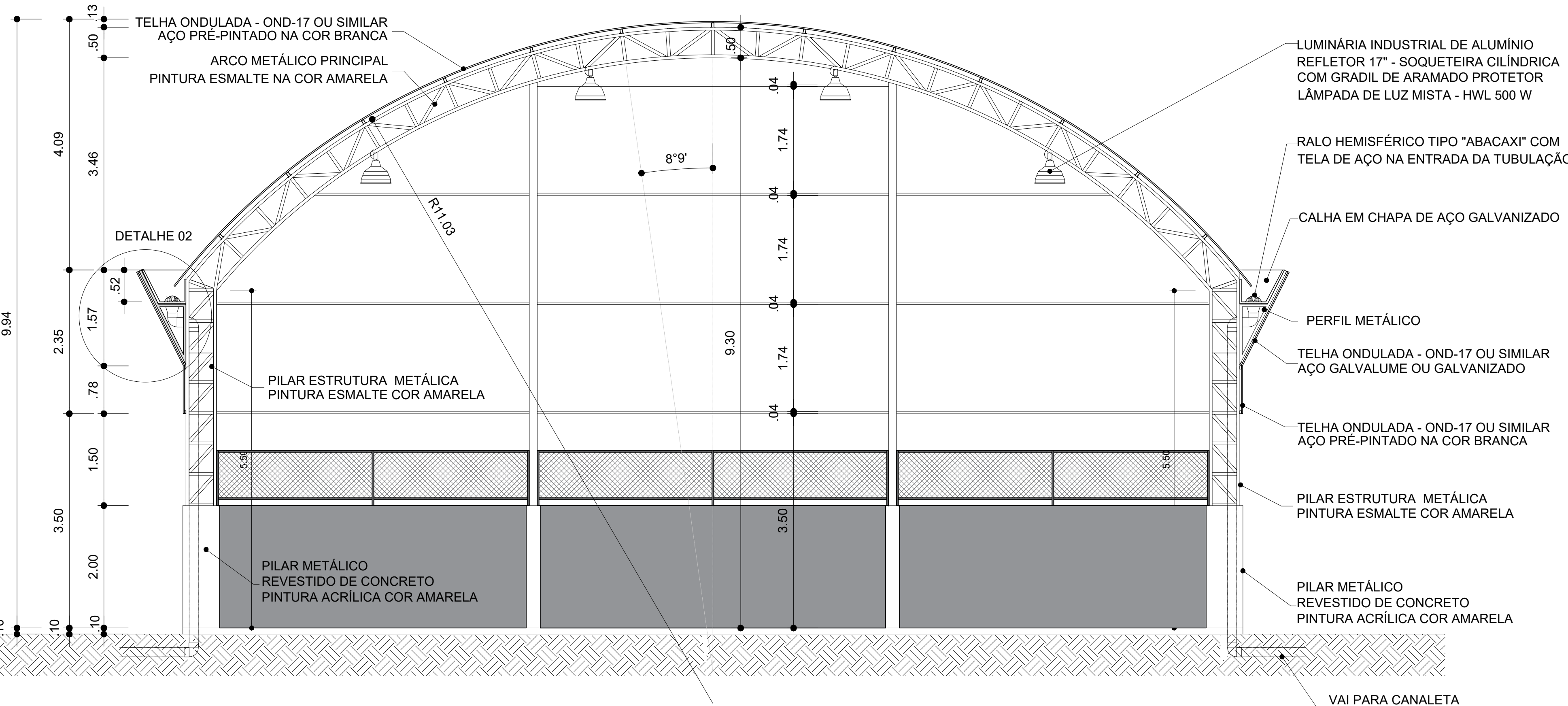
6 CORTE BB 1:50
