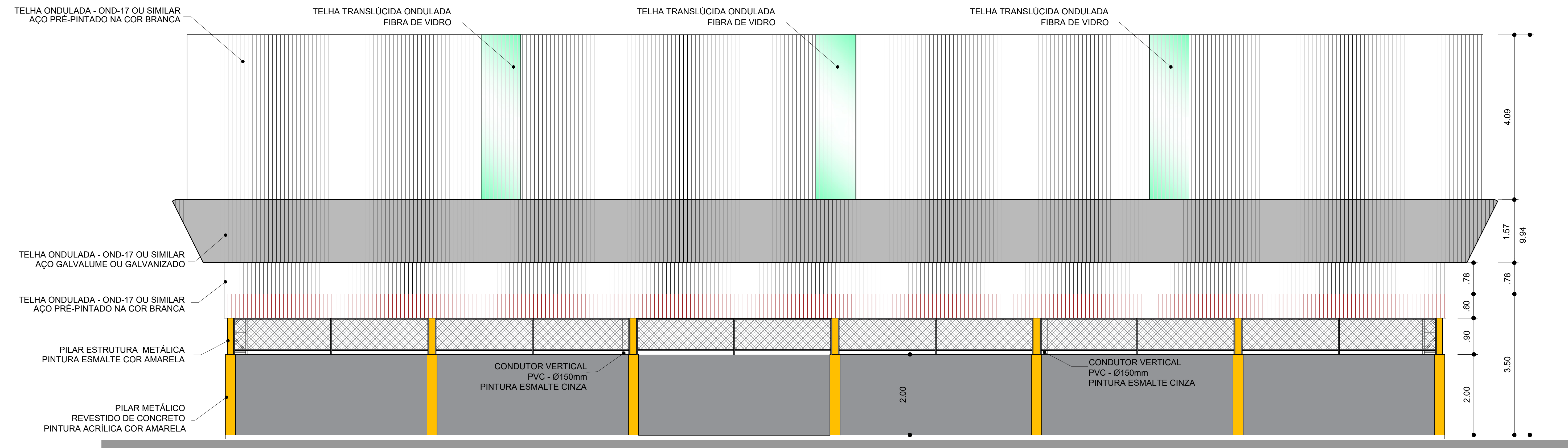
9 ELEVÇÃO 1 1:50
