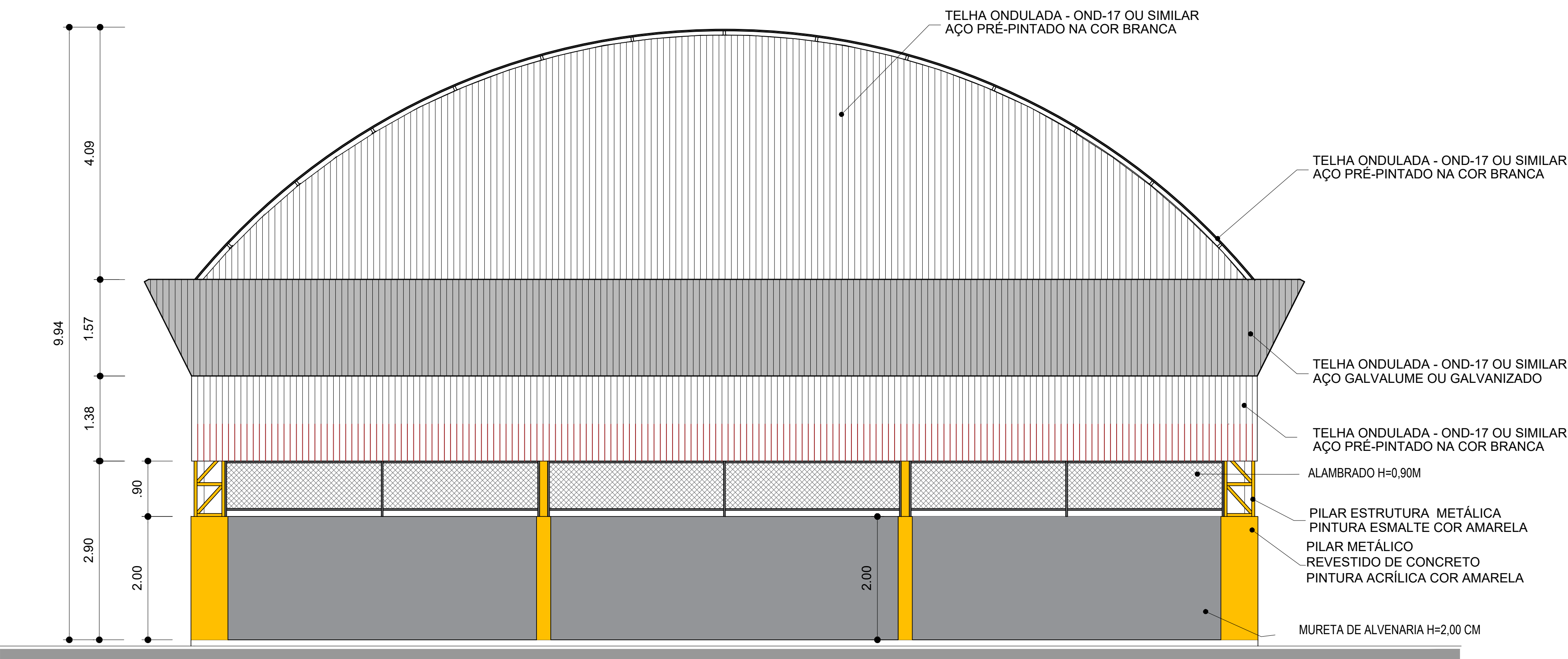
10 ELEVÇÃO 2 1:50
