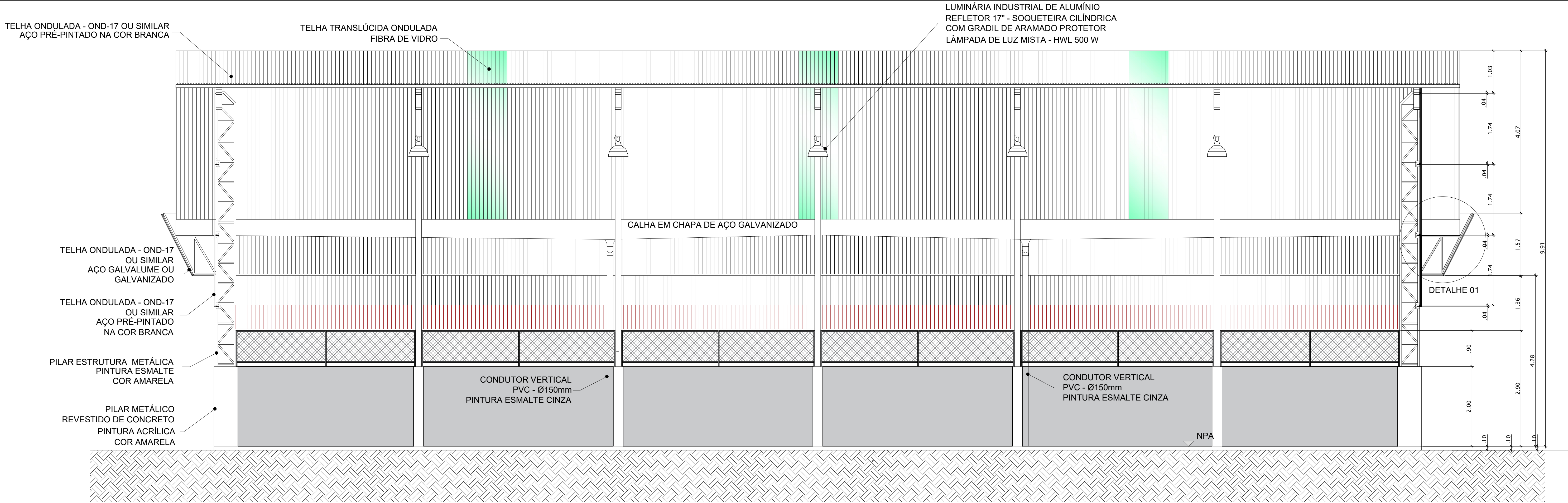
4 CORTE AA Esc.: 1 : 50
