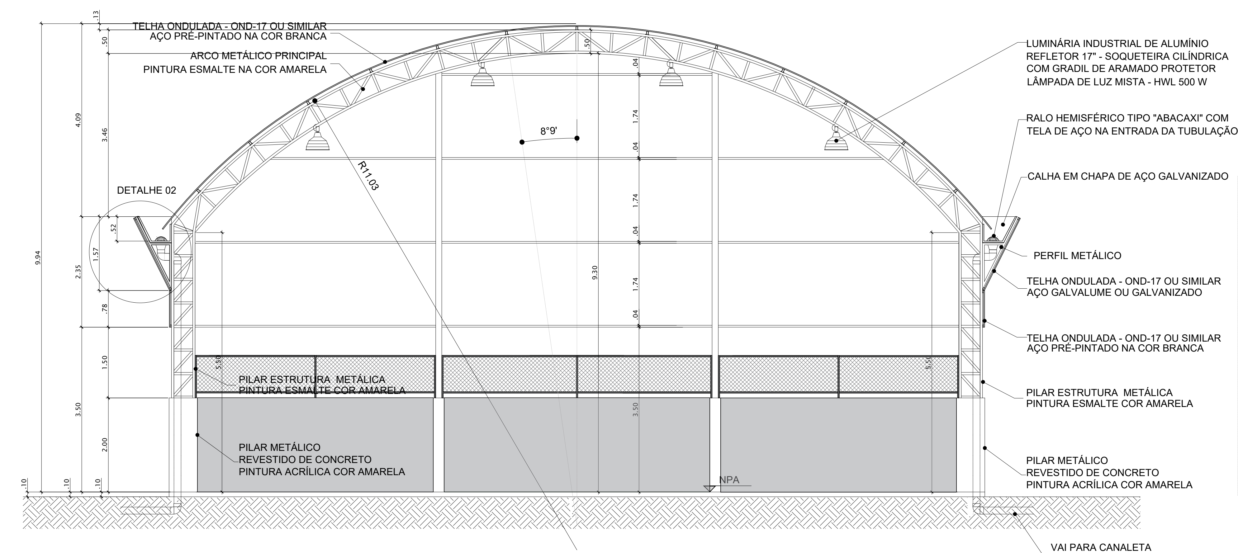
5 CORTE BB Esc.: 1 : 50
