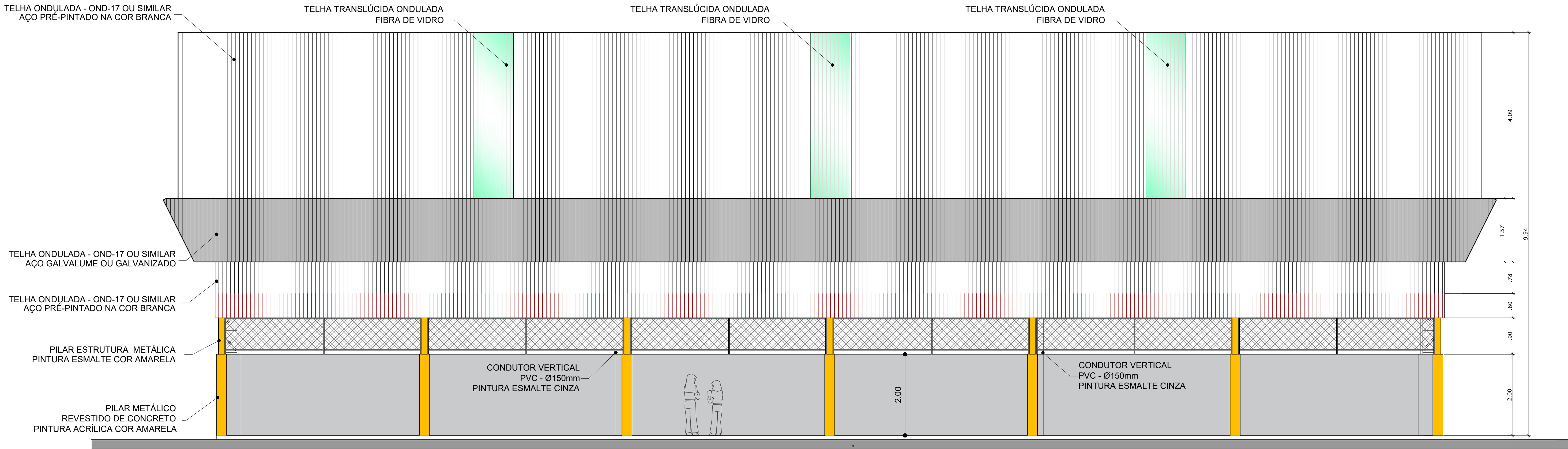
6 FACHADA 1 Esc.: 1 : 50
