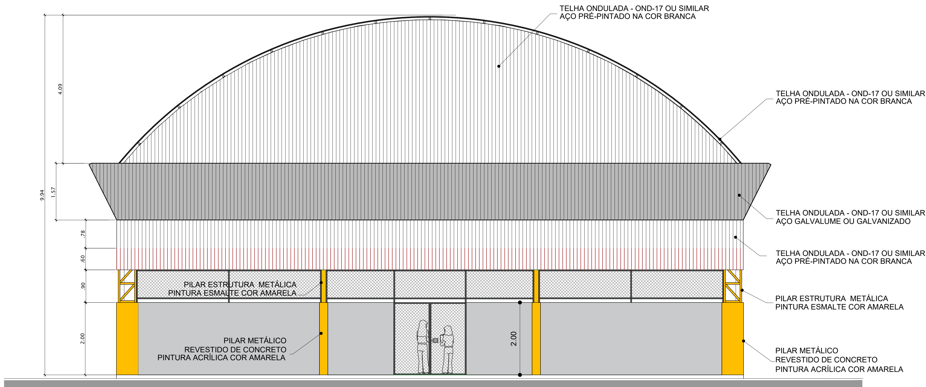
7 FACHADA 2 Esc.: 1 : 50
