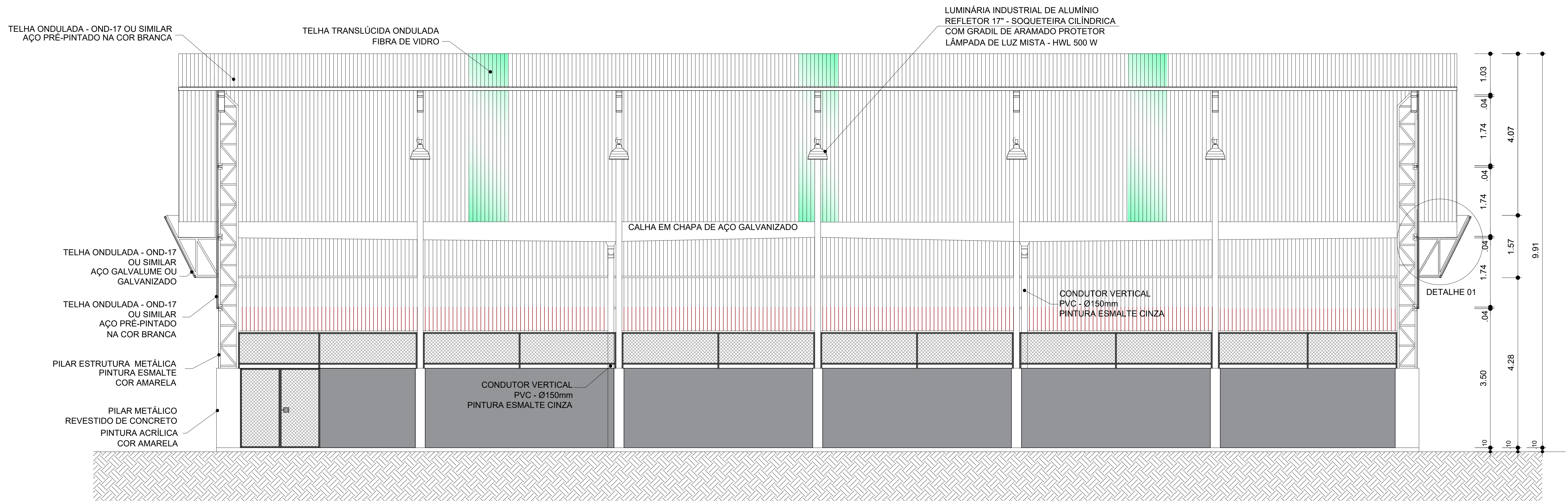
6 CORTE AA 1:50
