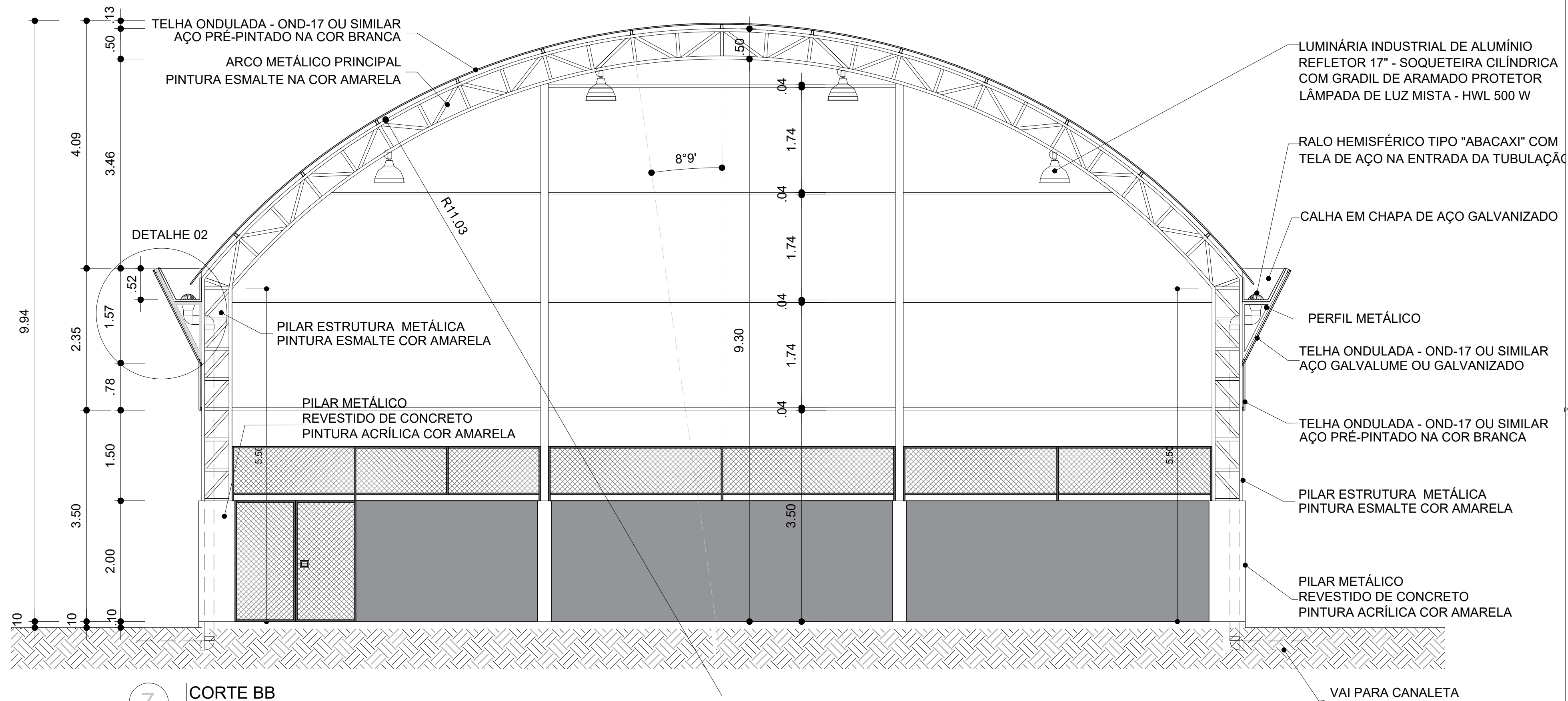
7 CORTE BB 1:50
