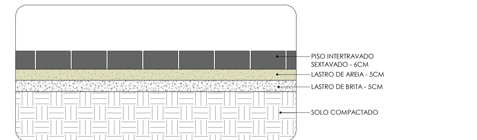
DET. PASSEIO INTERTRAVADO
