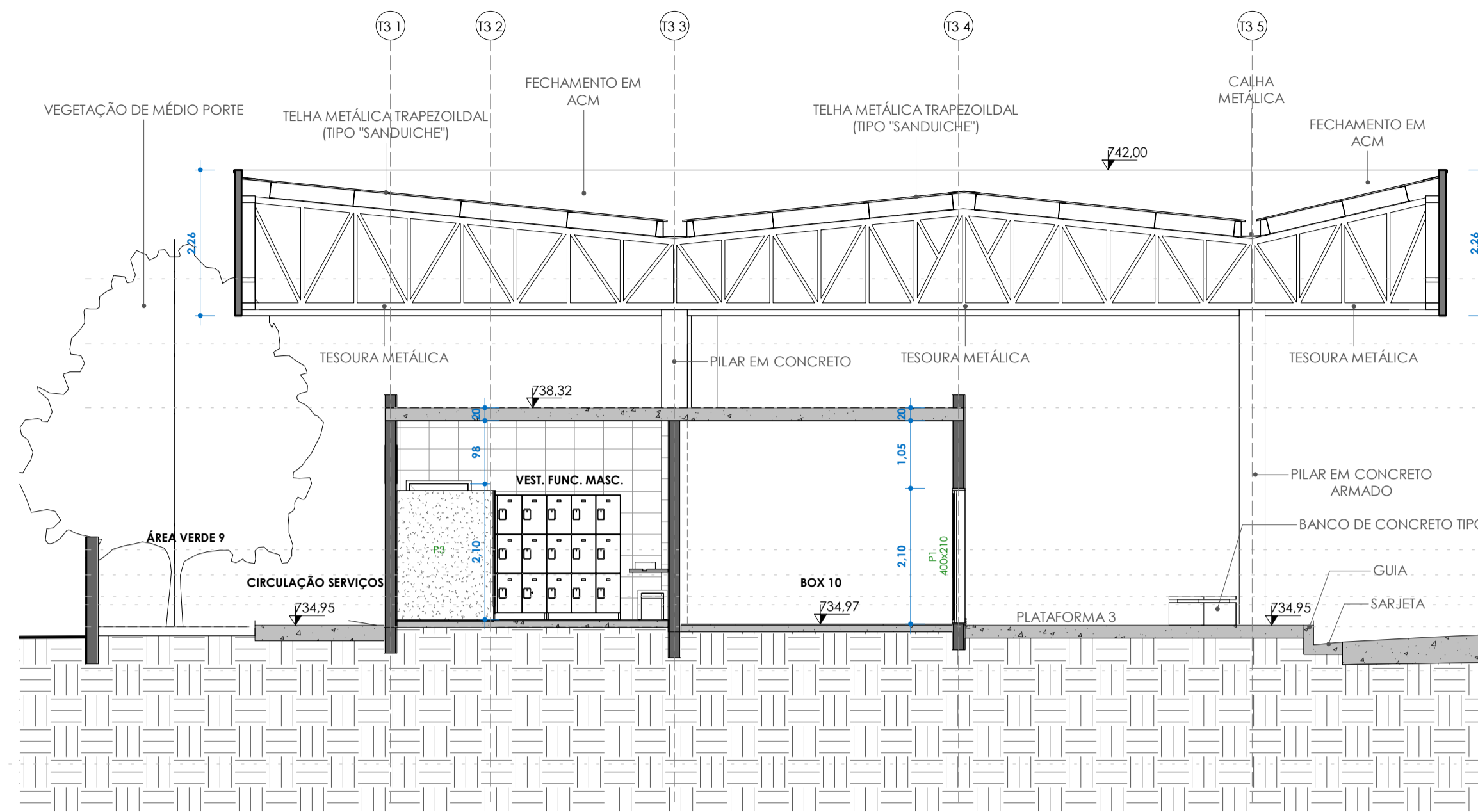
BB - PARTE 1/2 ESC:1 : 75
