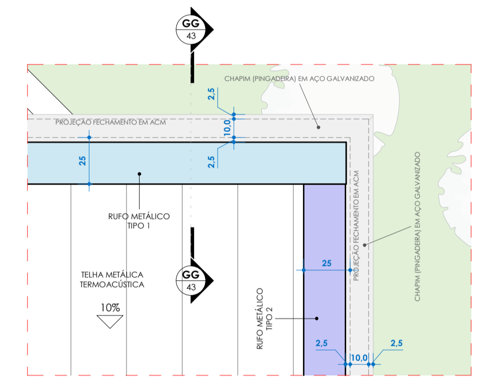
DETALHAMENTO - RUFO/PINGADEIRA ESC: 1 : 20 COTAS EM CENTÍMETROS
