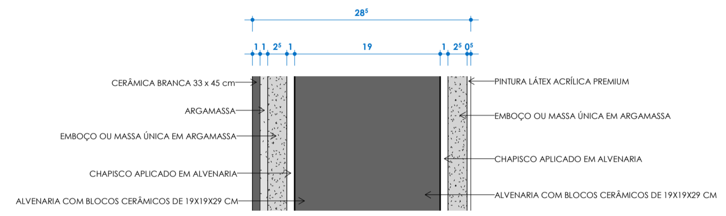
DET. PAREDE PINTURA/CERÂMICA ESC: 1 : 5
