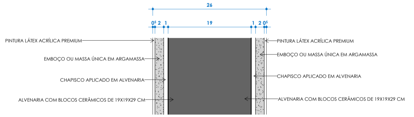
DET. PAREDE PINTURA/PINTURA ESC: 1 : 5
