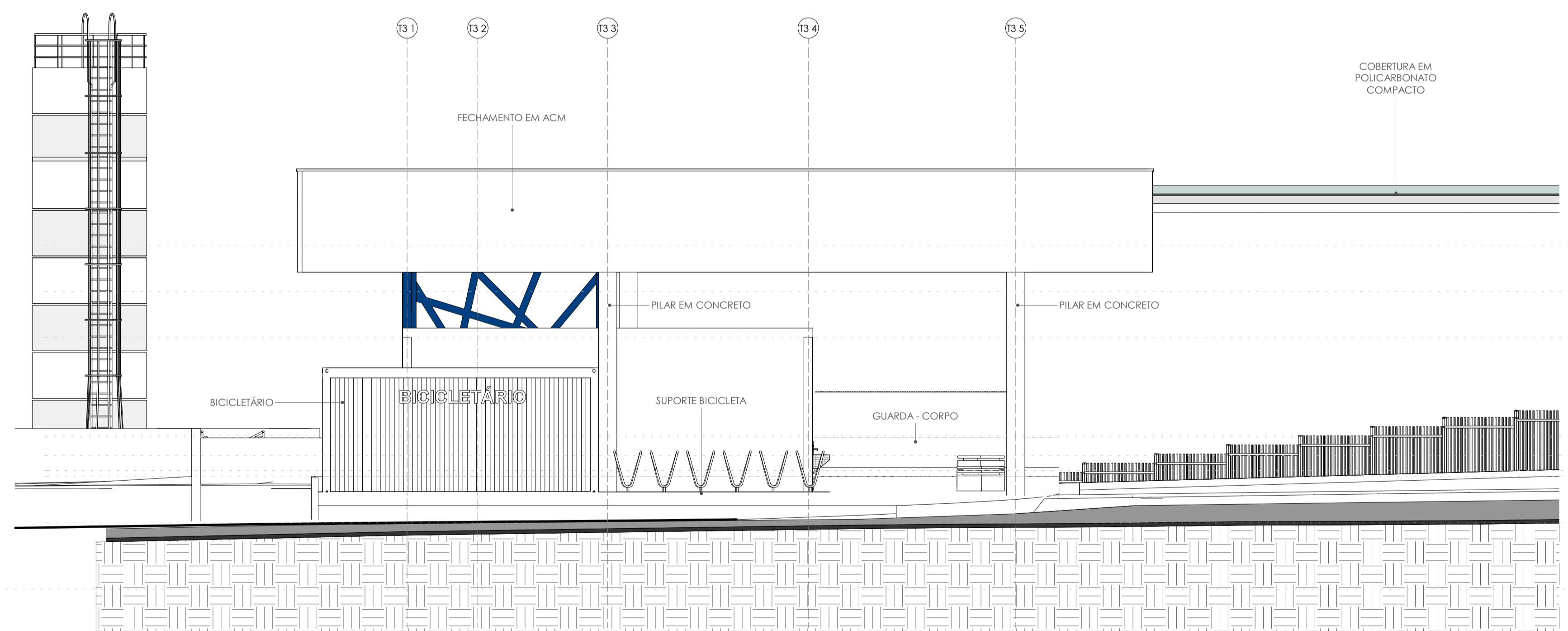
ELEVAÇÃO 3 - PARTE 1 ESC.: 1 : 75
