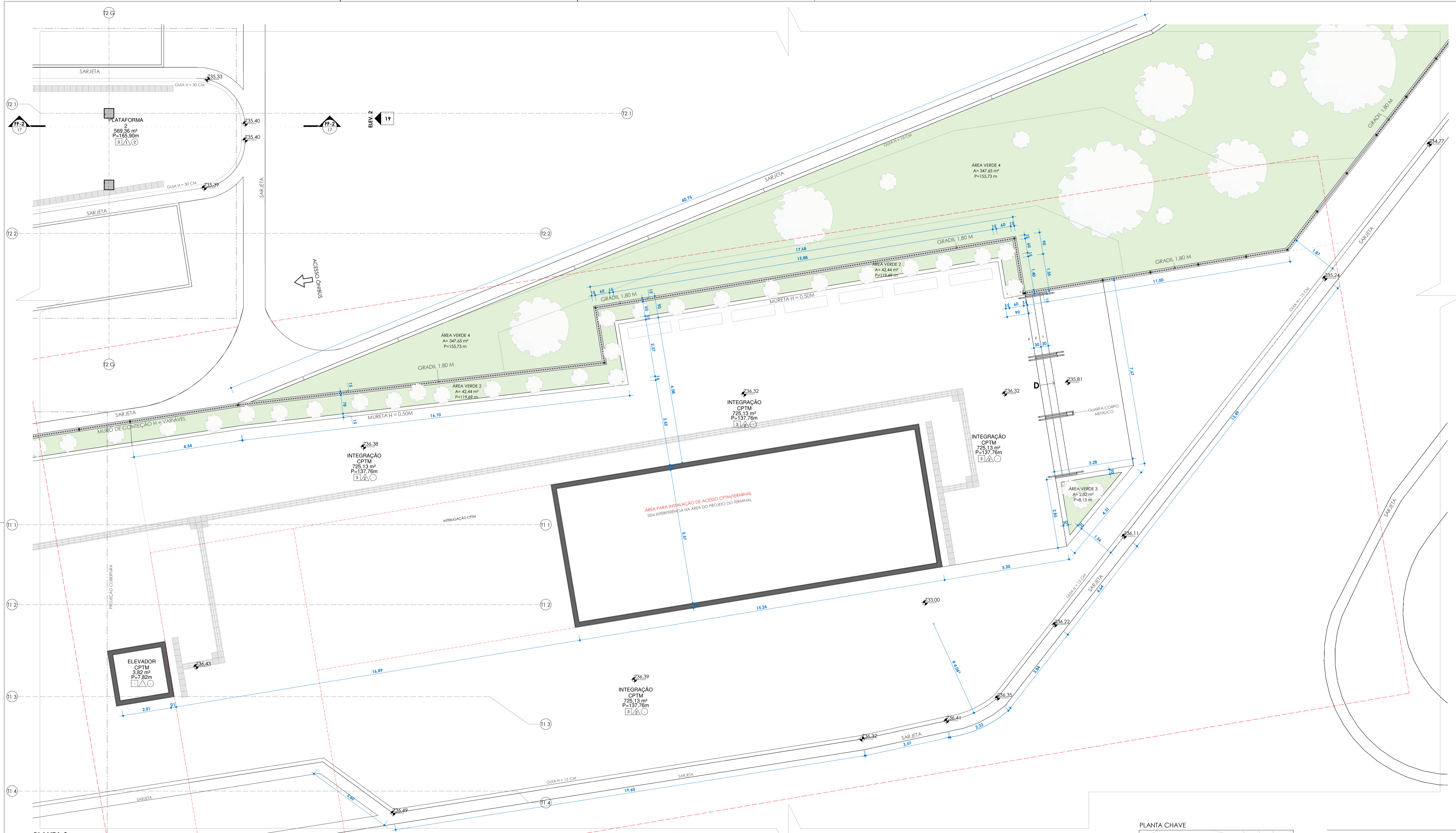
PLANTA 8 ESC: 1 : 75
