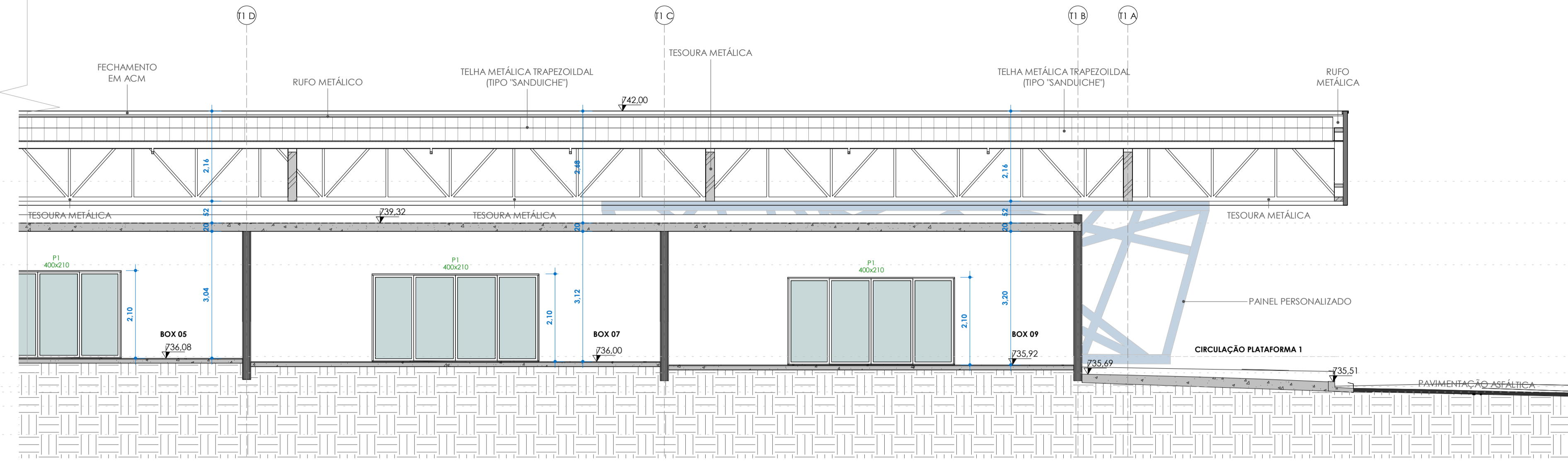
CC - PARTE 3 ESC:1 : 75
