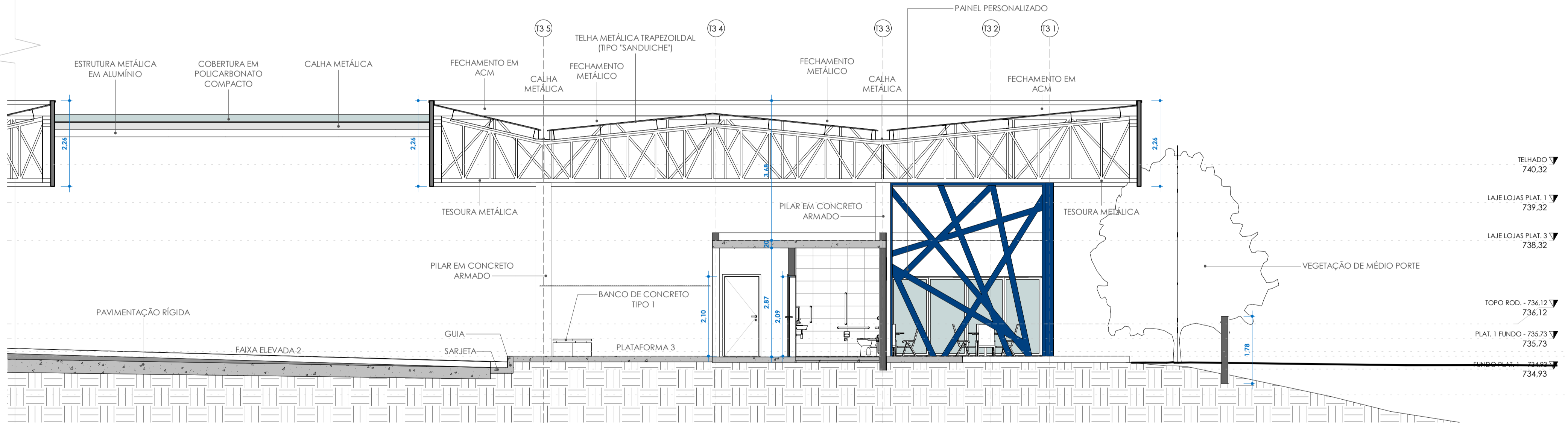
AA - PARTE 2/2 ESC: 1 : 75
