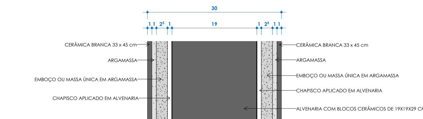
DET. PAREDE CERÂMICA/CERÂMICA ESC: 1 : 5
