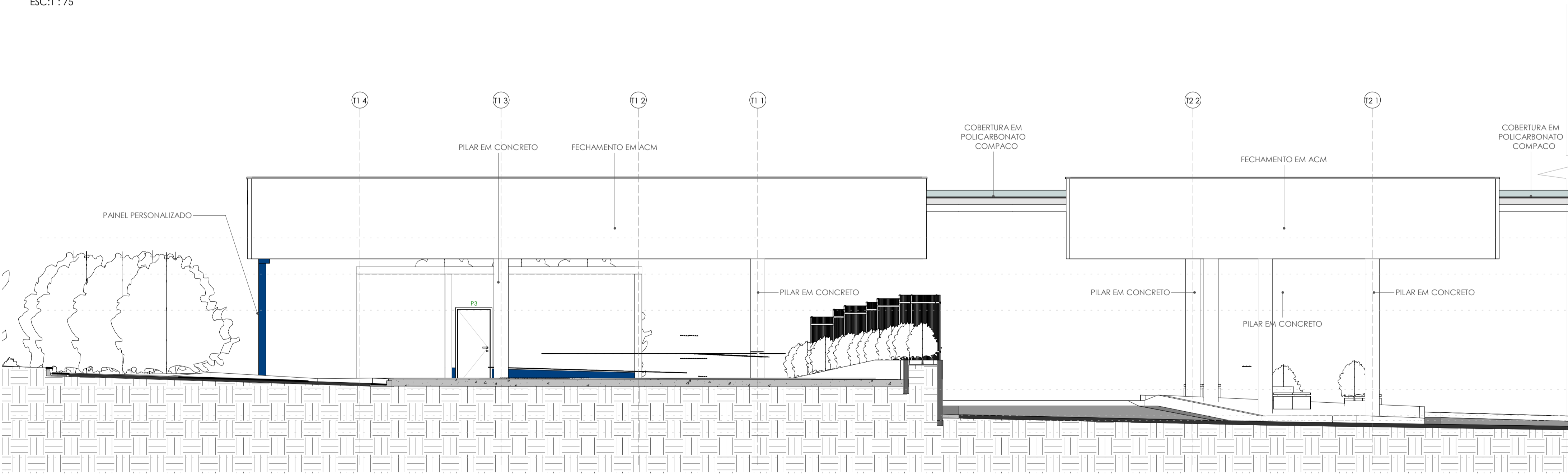
ELEVAÇÃO 2 - PARTE 1 ESC:1 : 75
