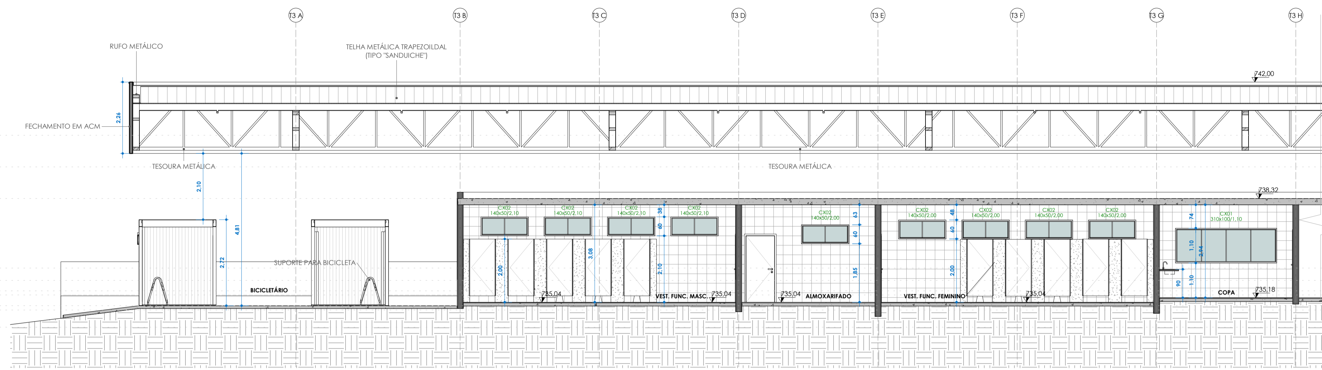
EE - PARTE 1/2 ESC:1 : 75
