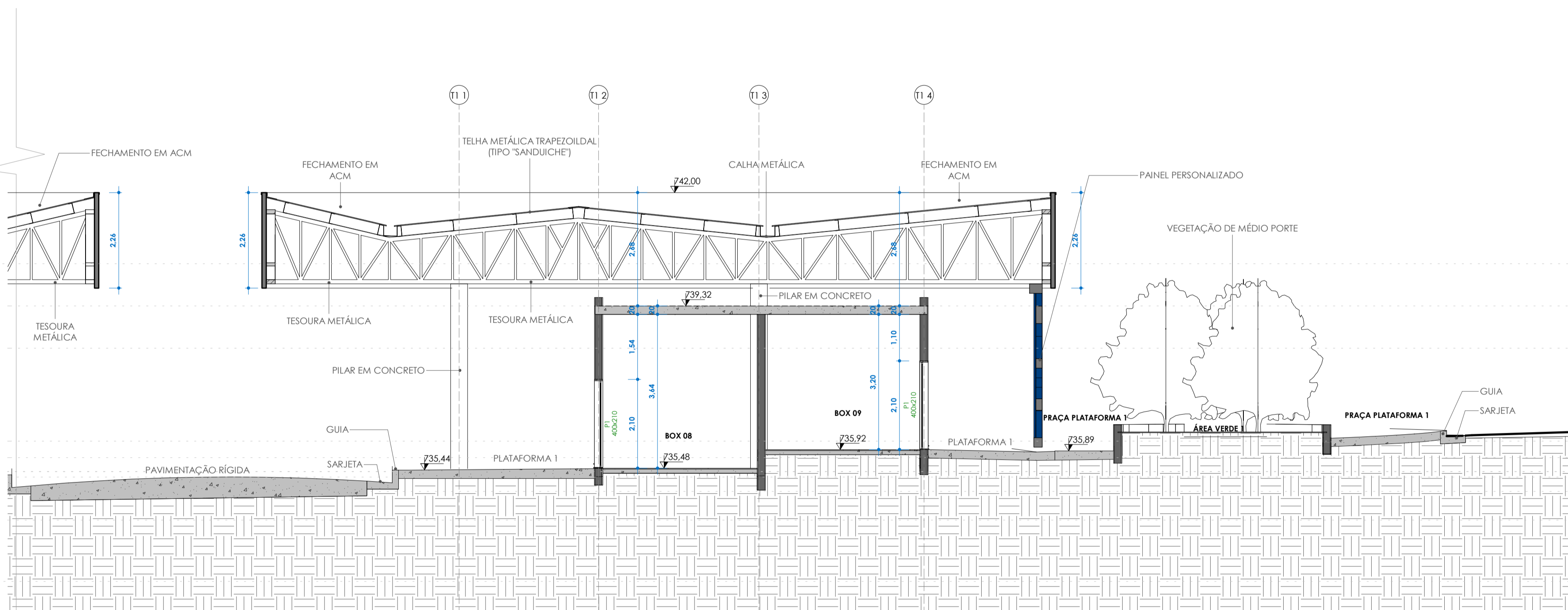
BB - PARTE 2/2 ESC:1 : 75
