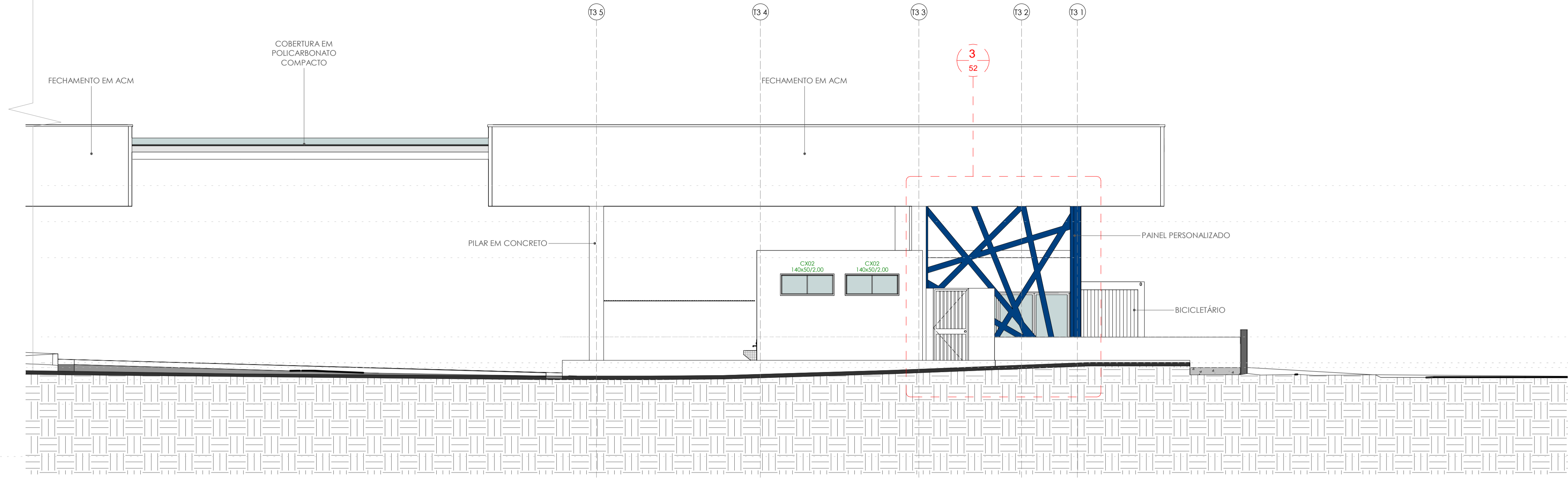
ELEVAÇÃO 2 - PARTE 2 ESC.: 1 : 75
