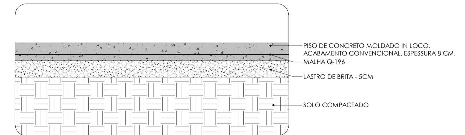
DET. PASSEIO DE CONCRETO
