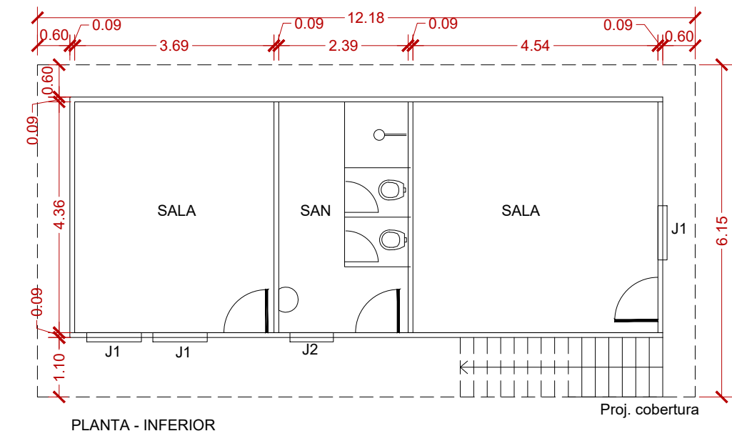
ALMOXARIFADO ESCALA - 1:100
