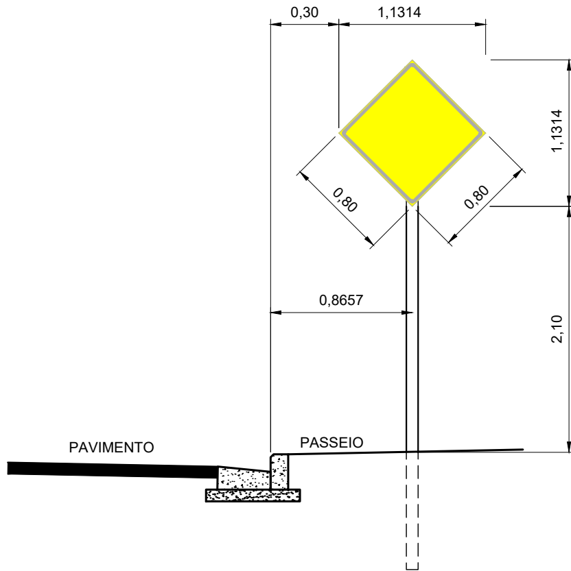
POSTE SIMPLES ADVERTÊNCIA S/ ESCALA
