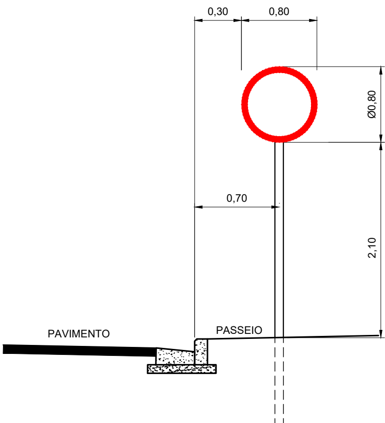
POSTE SIMPLES REGULAMENTAÇÃO S/ ESCALA
