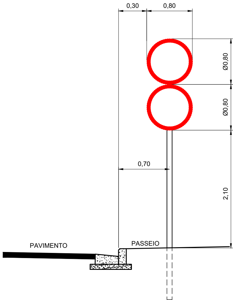
POSTE SIMPLES REGULAMENTAÇÃO C/ 2 PLACAS S/ ESCALA
