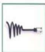
PONTA SEM FIM P-4 \varnothing 1" - 1 \frac{1}{2}" - 2" - 2 \frac{1}{2}" - 3" - 4" Utilizada em entupimentos com pano, estopa, papel, etc.
