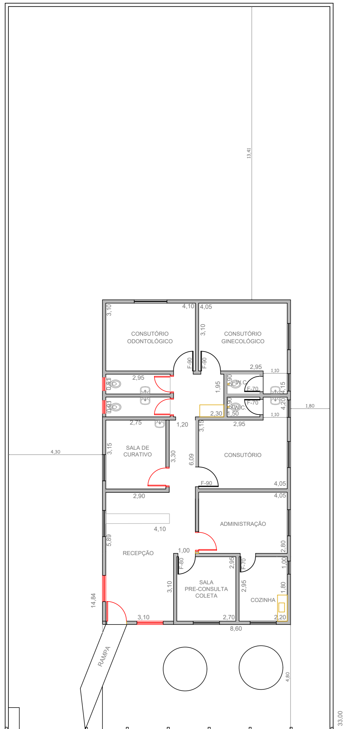
PLANTA BAIXA ESC 1:100
