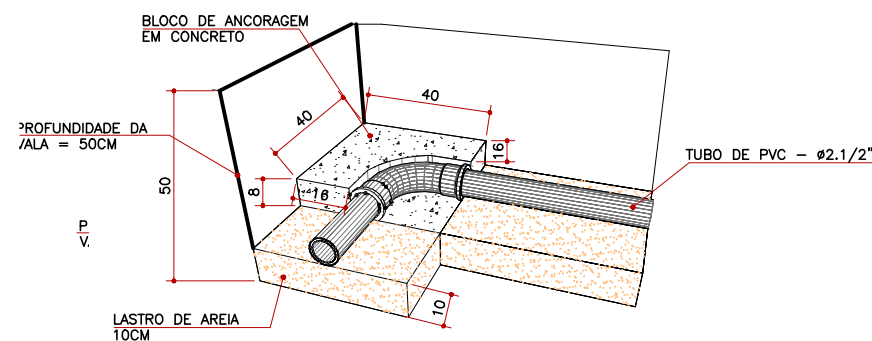
Detalhe em perspectiva - Bloco de Ancoragem em mudanças de direção SITUAÇÃO SEM ESCALA
