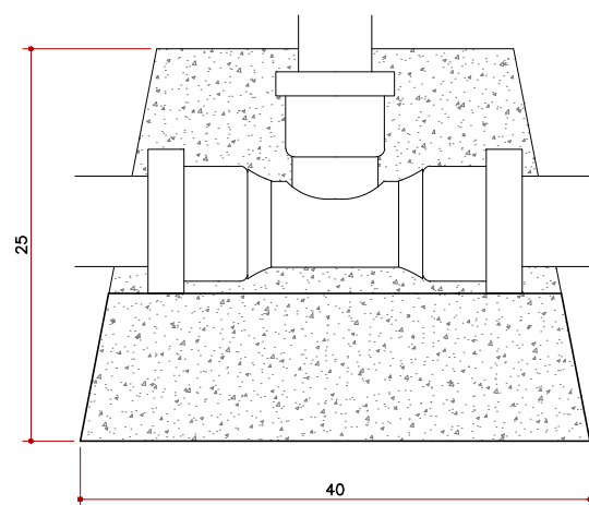
Detalhe em planta - Bloco de Ancoragem Conexão Te SITUAÇÃO SEM ESCALA
