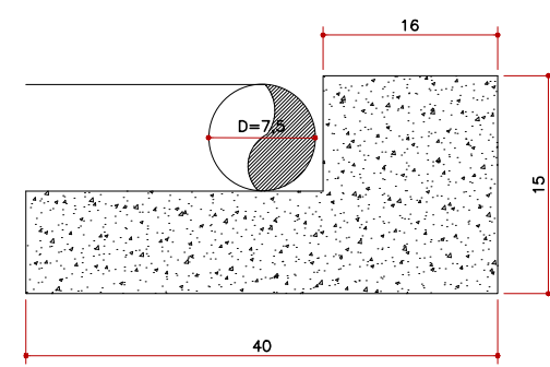
Detalhe em corte - Bloco de Ancoragem SITUAÇÃO SEM ESCALA
