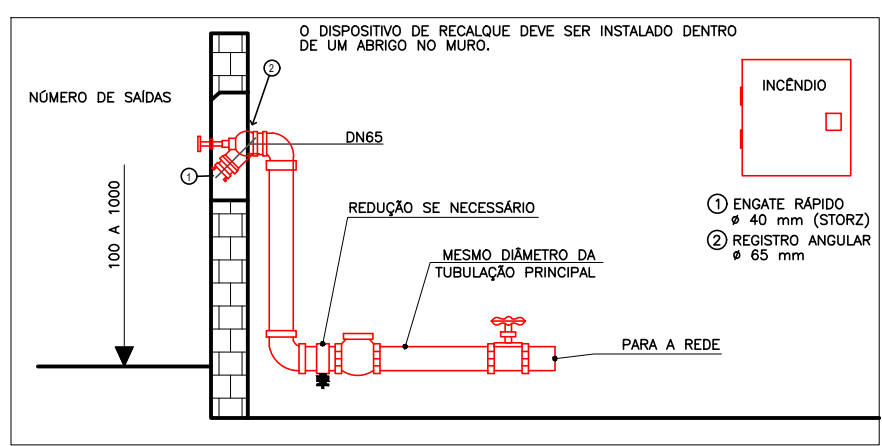
DISPOSITIVO DE RECALQUE TIPO COLUNA SITUAÇÃO SEM ESCALA
