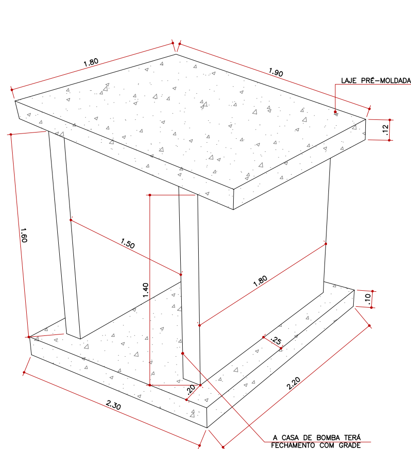
Perspectiva Casa de Bomba SITUAÇÃO SEM ESCALA
