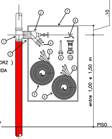
DETALHE DO QUADRO DE SINALIZAÇÃO SITUAÇÃO SEM ESCALA
