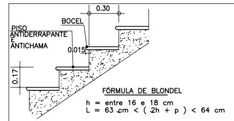
DETALHE DO ESCADA SITUAÇÃO SEM ESCALA
