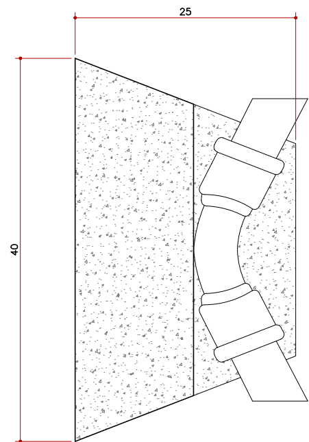
Detalhe em planta - Bloco de Ancoragem Curva SITUAÇÃO SEM ESCALA
