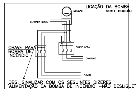
ESQUEMA DE ALIMENTAÇÃO ELÉTRICA DA BOMBA DE INCÊNDIO SITUAÇÃO SEM ESCALA
