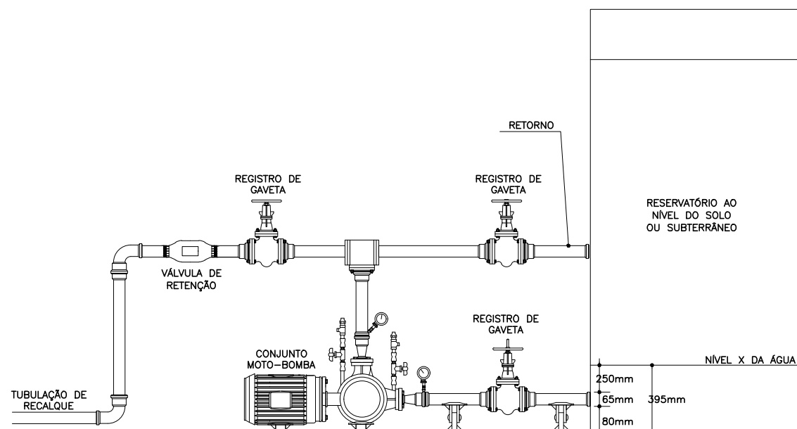
DETALHE CONJUNTO MOTO-BOMBA SITUAÇÃO SEM ESCALA
