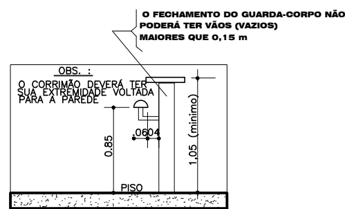
DETALHE DO CORRIMÃO SITUAÇÃO SEM ESCALA
