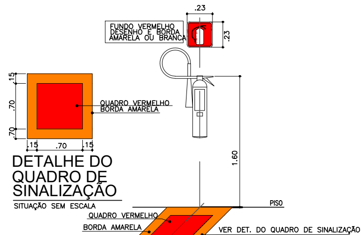
DETALHE DA SINALIZAÇÃO AÉREA E DE SOLO E ALTURA MÁXIMA DOS EXTINTORES SITUAÇÃO SEM ESCALA
