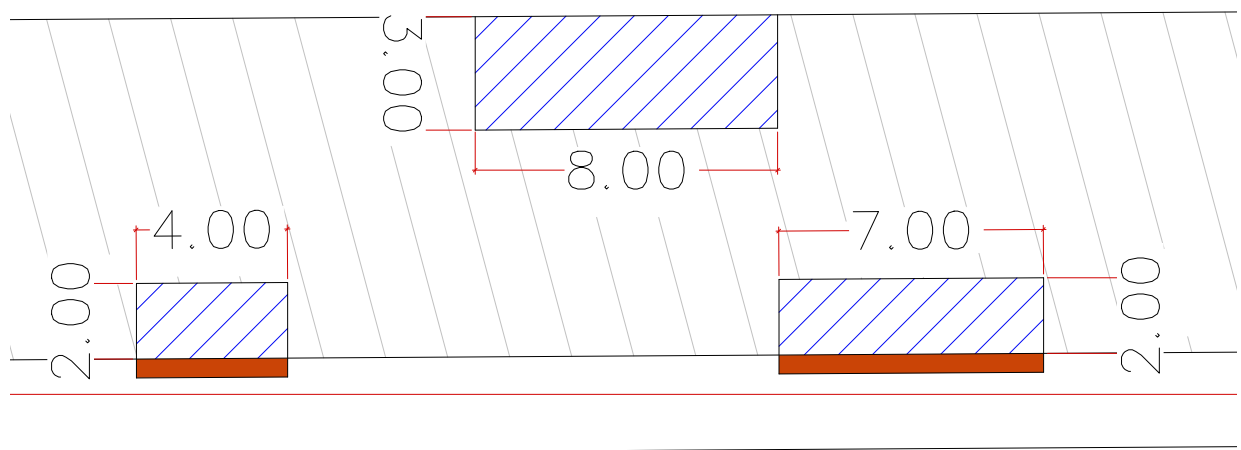
Detalhe 02 Escala 1:100
