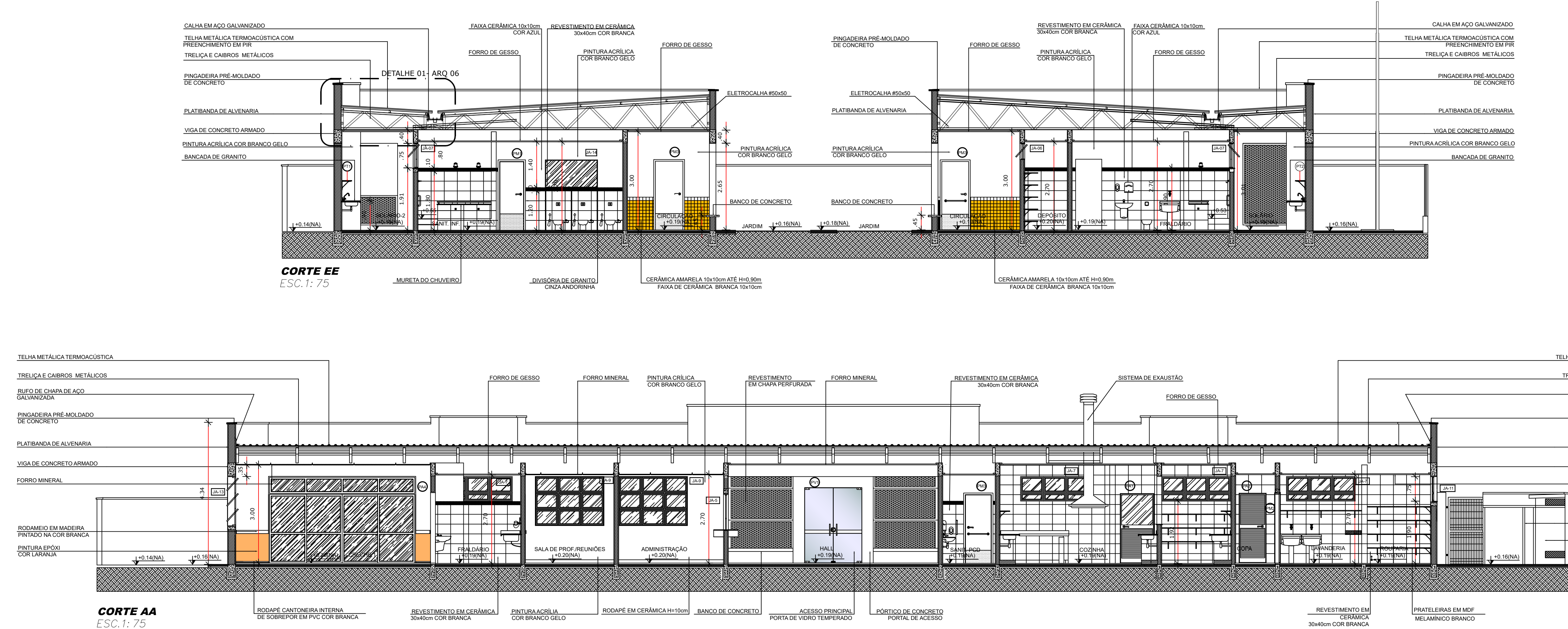
CORTE AA ESC: 1:75
