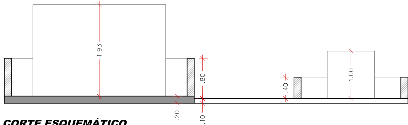
CORTE ESQUEMÁTICO ESC. 1: 50
