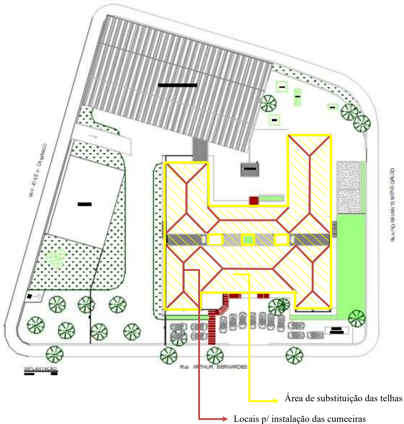
IMAGEM 1 SUBSTITUIÇÃO DAS TELHAS E CUMEEIRAS
