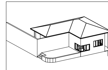
4 VISTA ISOMÉTRICA
