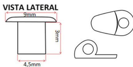
Figura 14 - Ilhós Redondo Latão 51 e Ilhós Gancho Zamac
