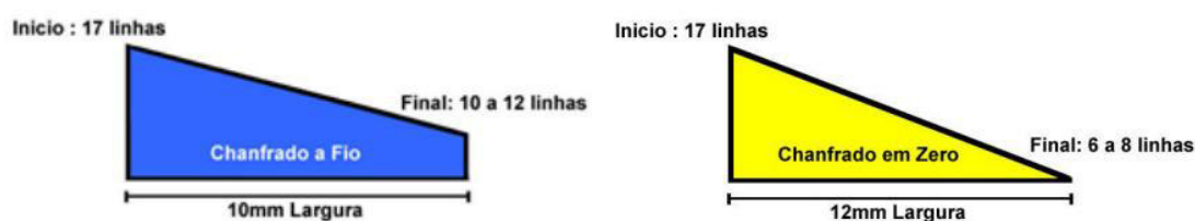
Figura 2 - Informações do Chanfro
