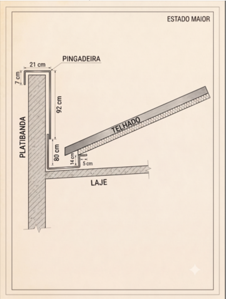
B) Sistema de Rufos e Pingadeiras Laterais de ambos os prédios:
