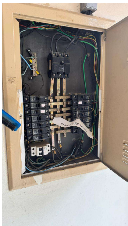
Figura 3 - Quadro de disjuntor - Depósito terceirizados lado direito
