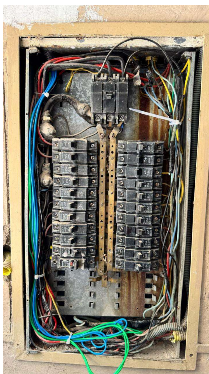
Figura 2 - Quadro de disjuntor - Depósito NPE
