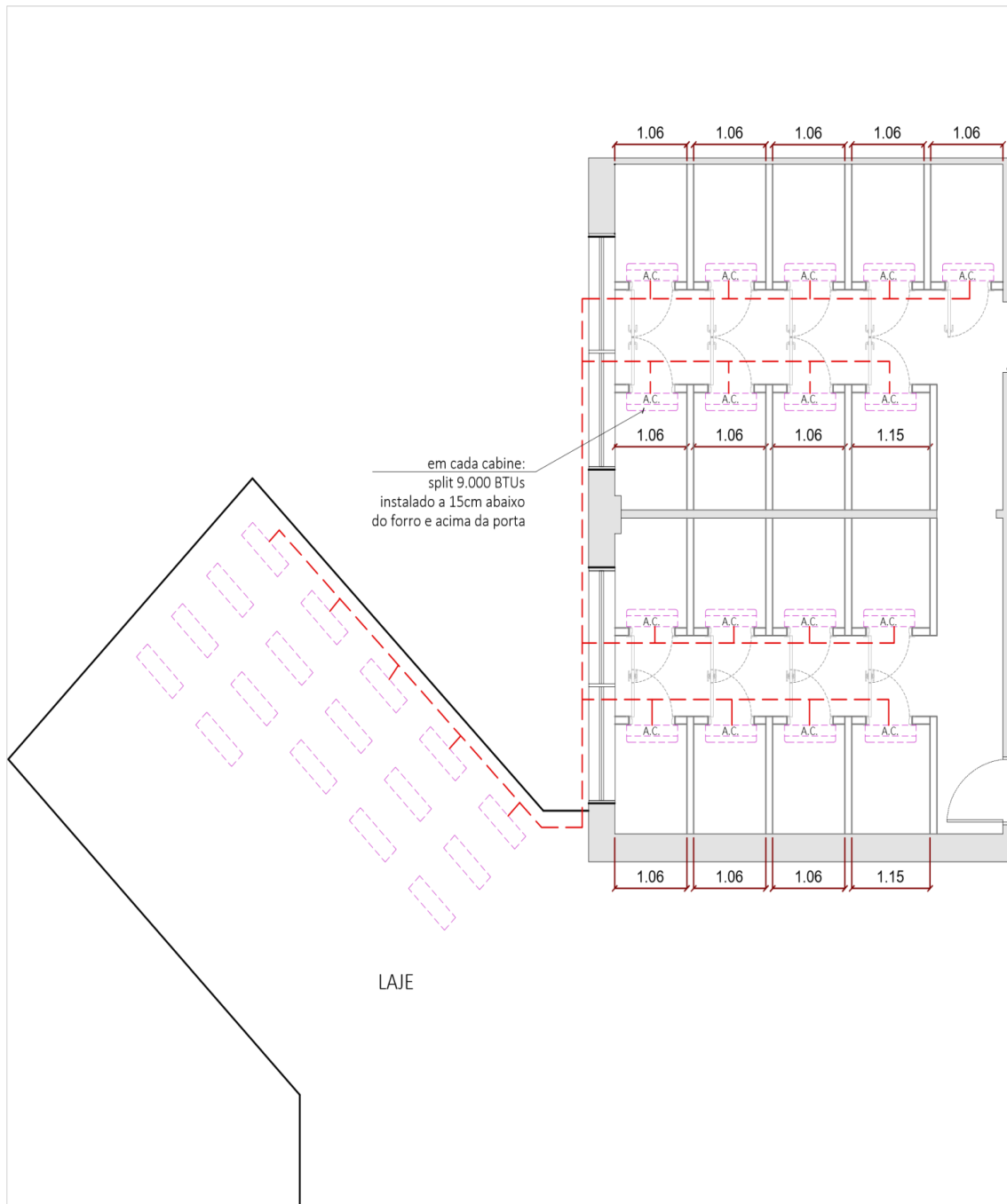
PLANTA LOCALIZAÇÃO DE CONDENSADORAS ESC. 1:75
