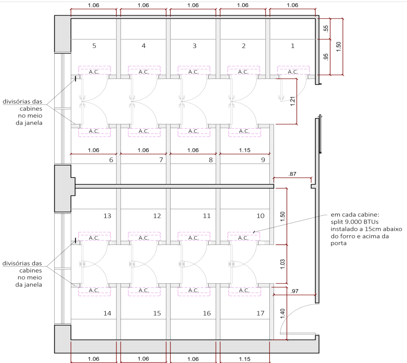
PLANTA TÉCNICA COM COTAS - ESTUDO ESC. 1:50
