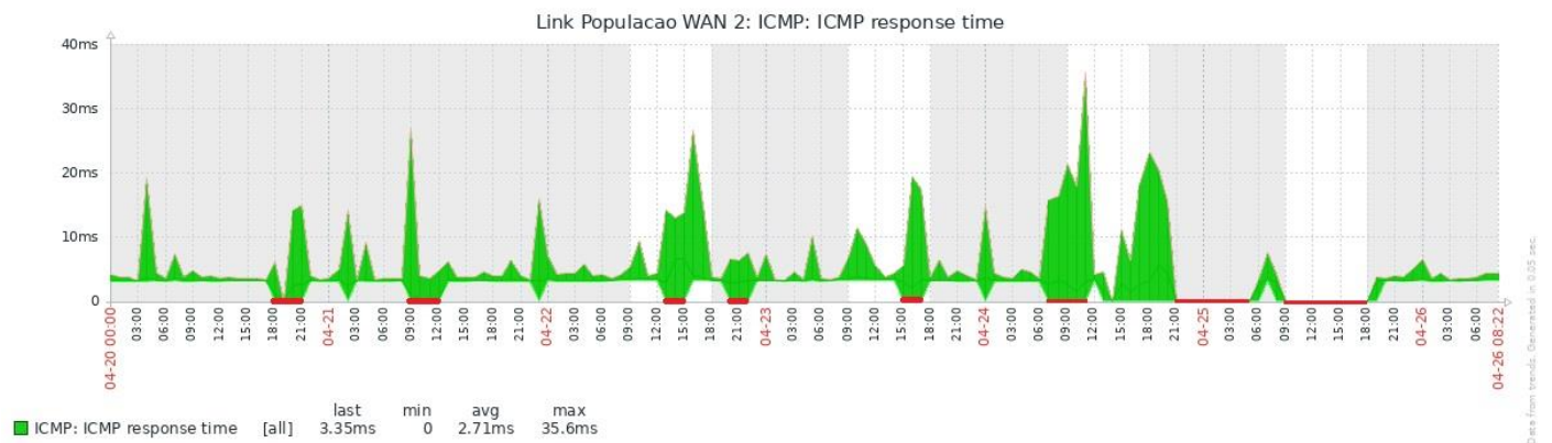
FIGURA 12 – Tempo de indisponibilidade do link de 500Mbps.
