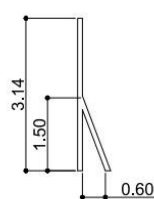
04 Detalhes dos "postes" de sustentação Esc. 1:50
