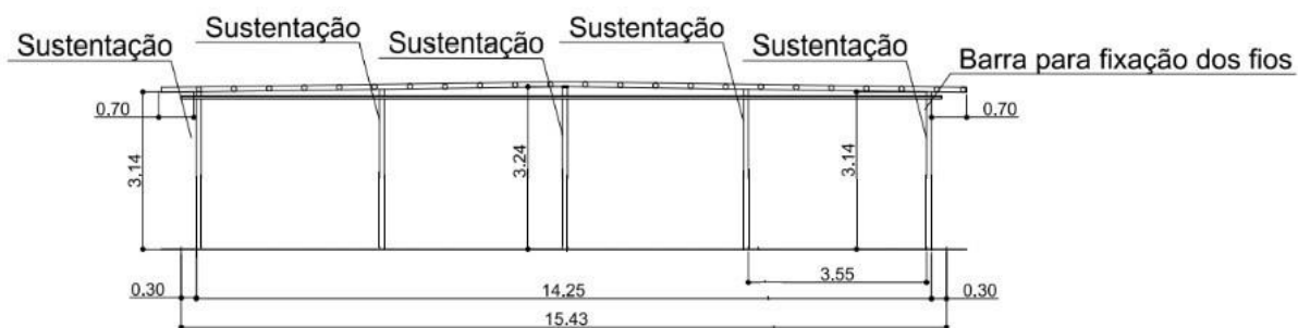
03 Vista lateral Esc. 1:75
