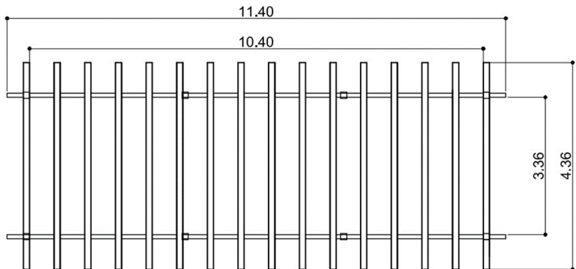
Figuras 11, 12 e 13 – Planta Baixa - Pergolados Laterais 01 e 02
