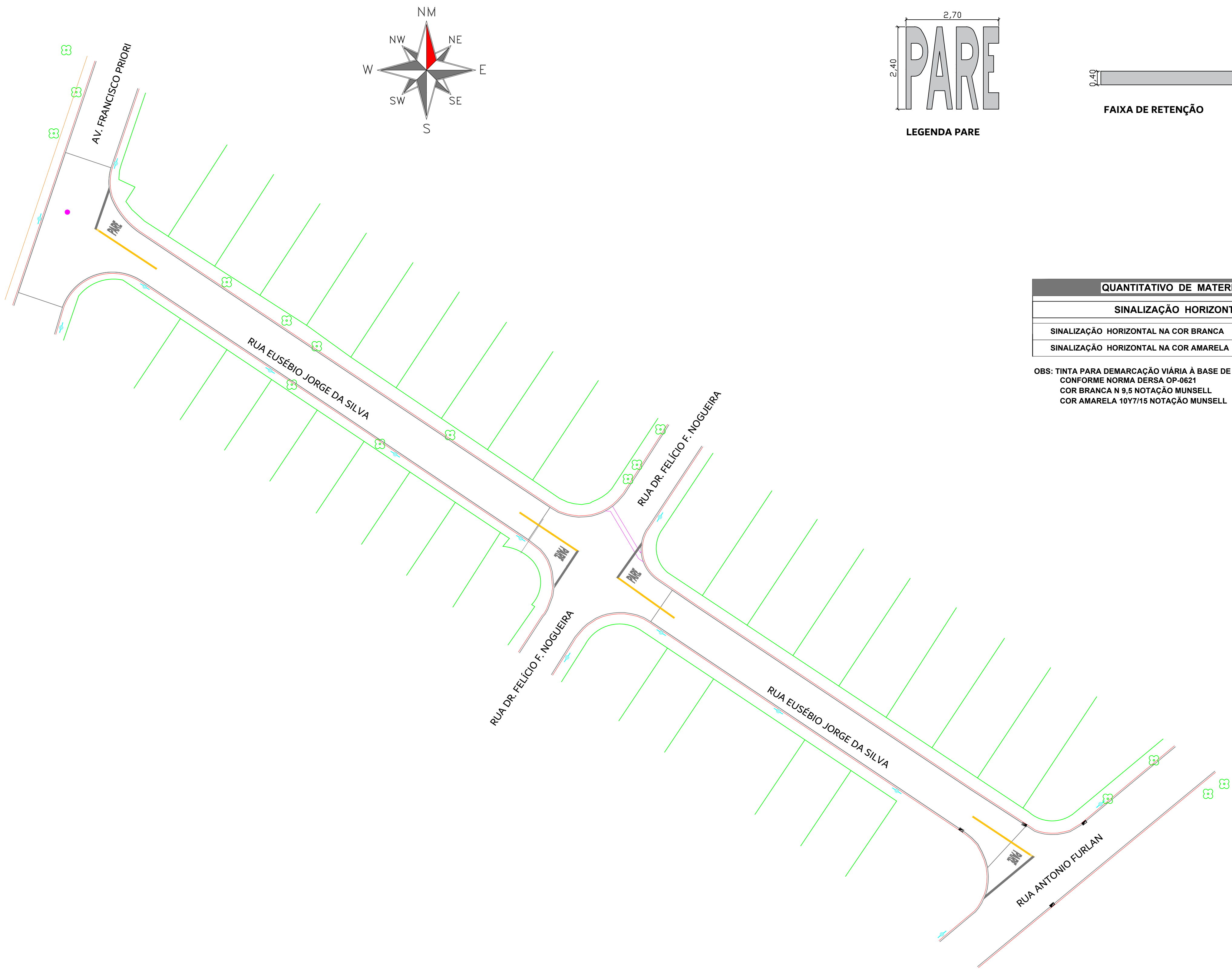
PLANTA DE LOCAÇÃO DA VIA ESCALA 1:500
