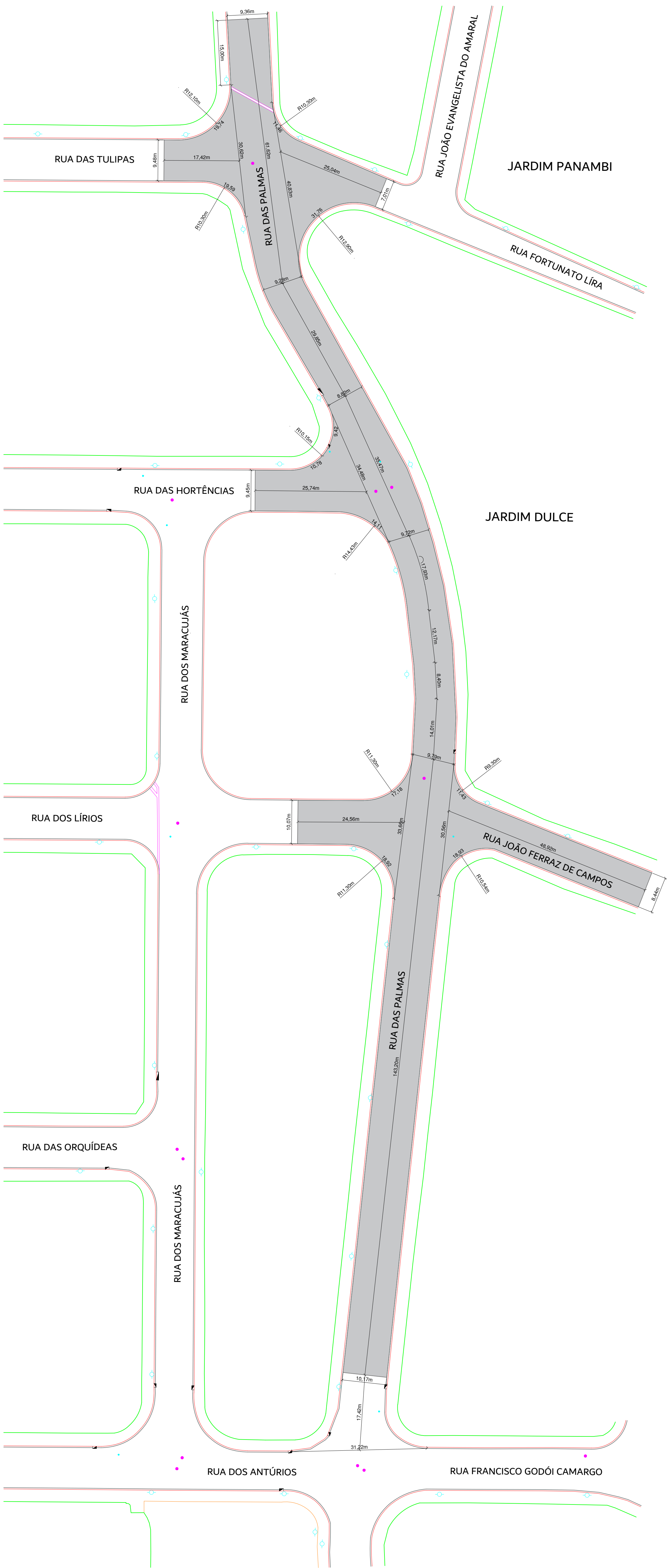
PLANTA DE LOCAÇÃO DA VIA - RUA DAS PALMAS ESCALA 1:500
