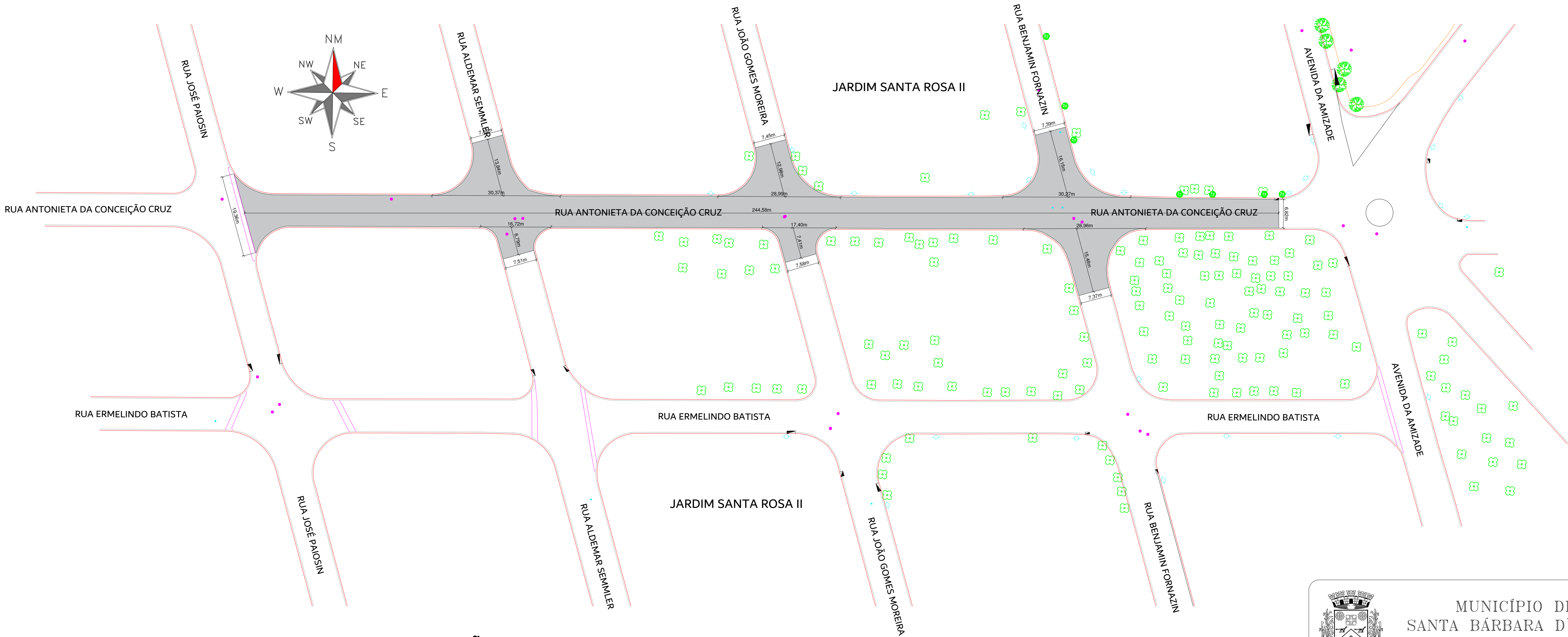
PLANTA DE LOCAÇÃO DA VIA ESCALA 1:500
