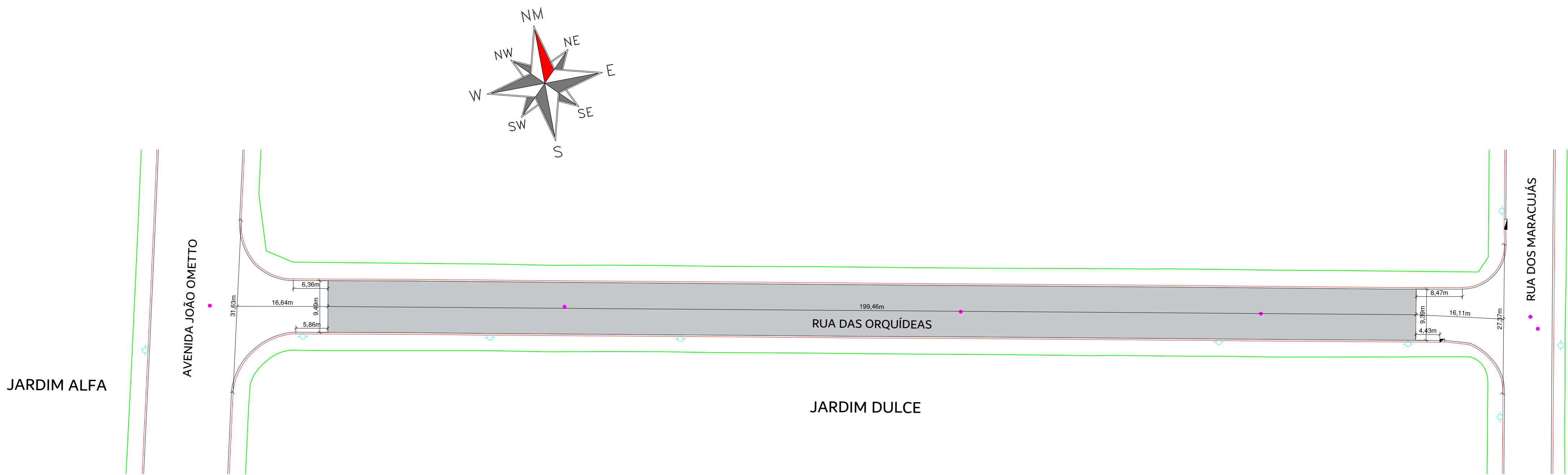
PLANTA DE LOCAÇÃO DA VIA - RUA DAS ORQUÍDEAS ESCALA 1:500
