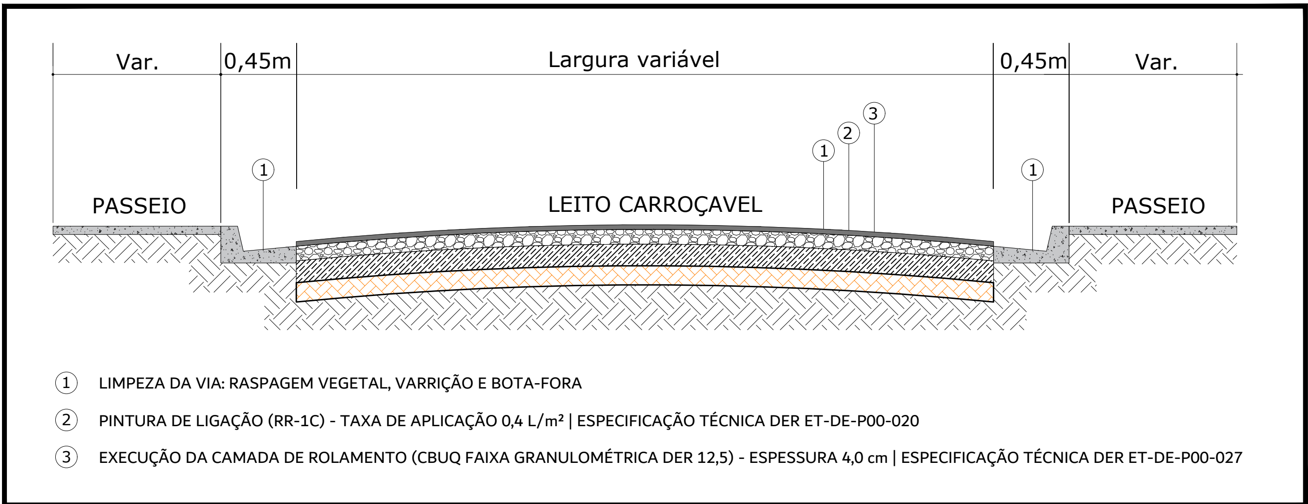
DETALHE CONSTRUTIVO - RECAPEAMENTO ASFÁLTICO SIMPLES SEM ESCALA
