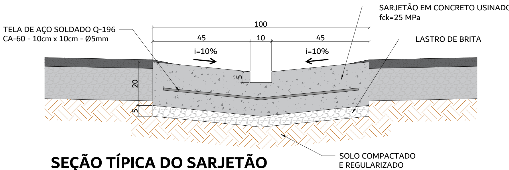
SEÇÃO TÍPICA DO SARJETÃO ESCALA 1:10
