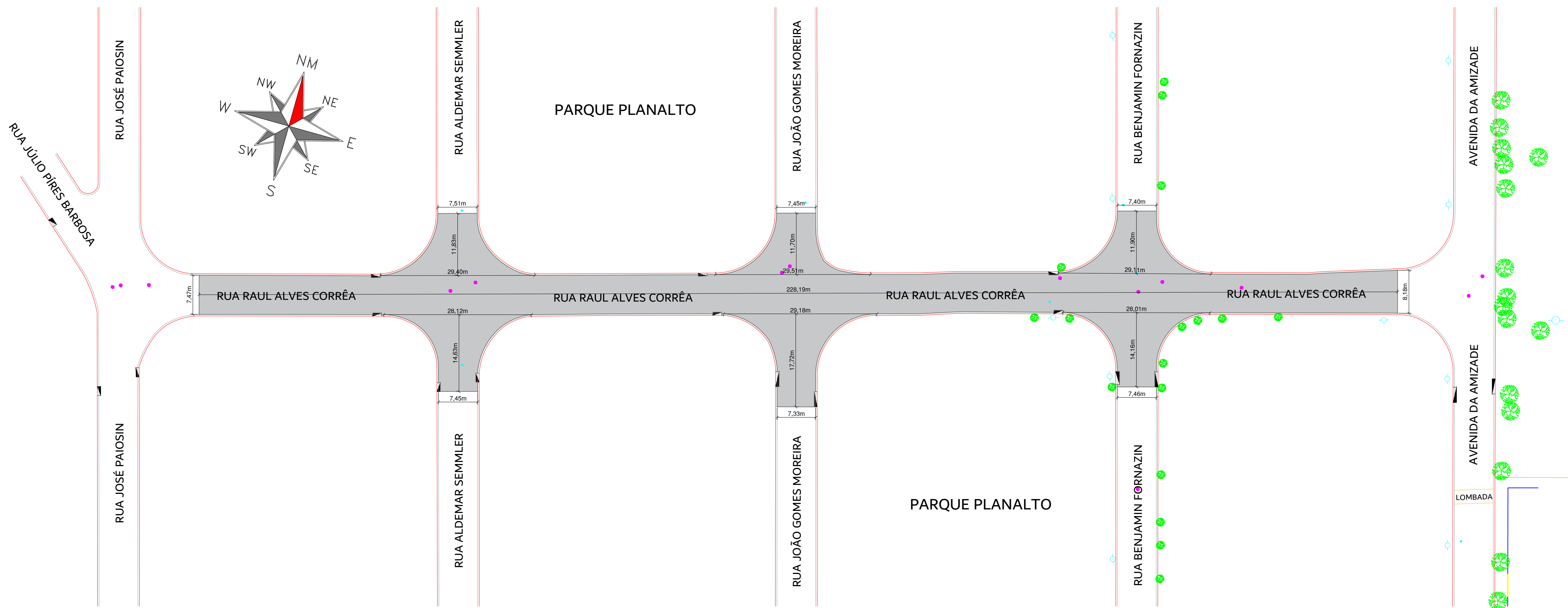
PLANTA DE LOCAÇÃO DA VIA ESCALA 1:500
