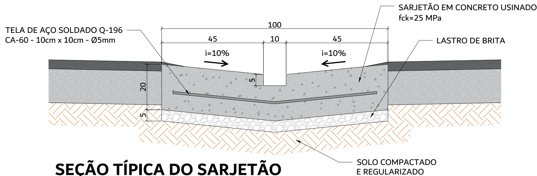
SEÇÃO TÍPICA DO SARJETÃO ESCALA 1:10
