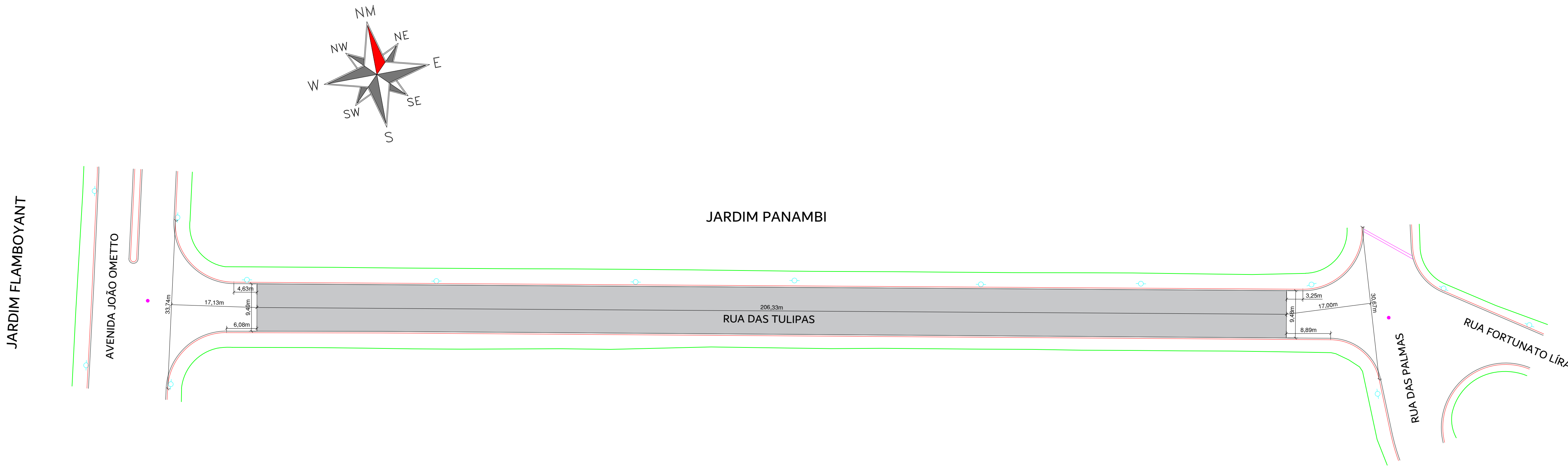
PLANTA DE LOCAÇÃO DA VIA - RUA DAS TULIPAS ESCALA 1:500
