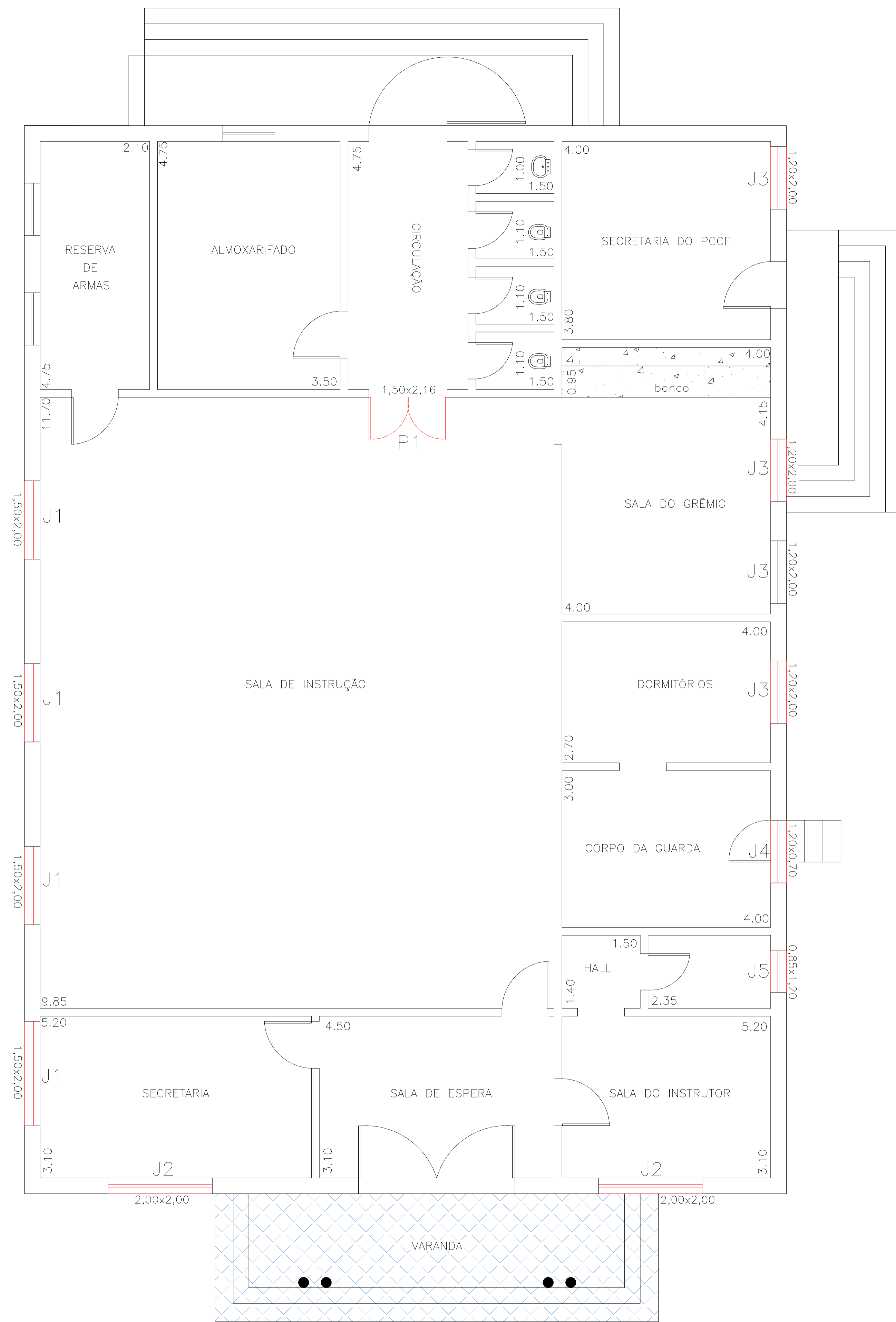
Planta Baixa ESCALA 1:50
