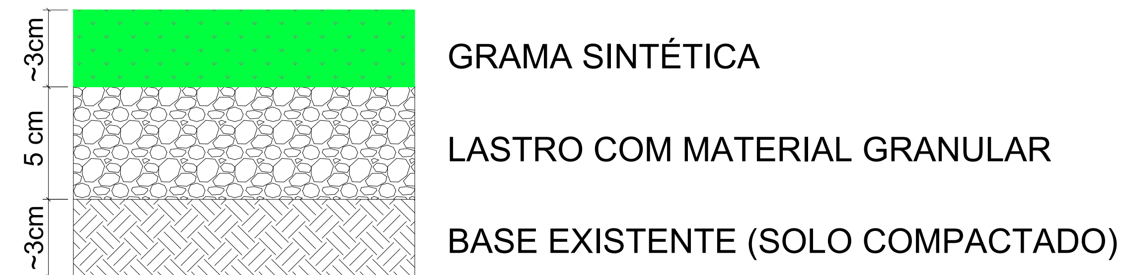
DETALHE INSTALAÇÃO DA GRAMA SINTÉTICA SEM ESCALA
