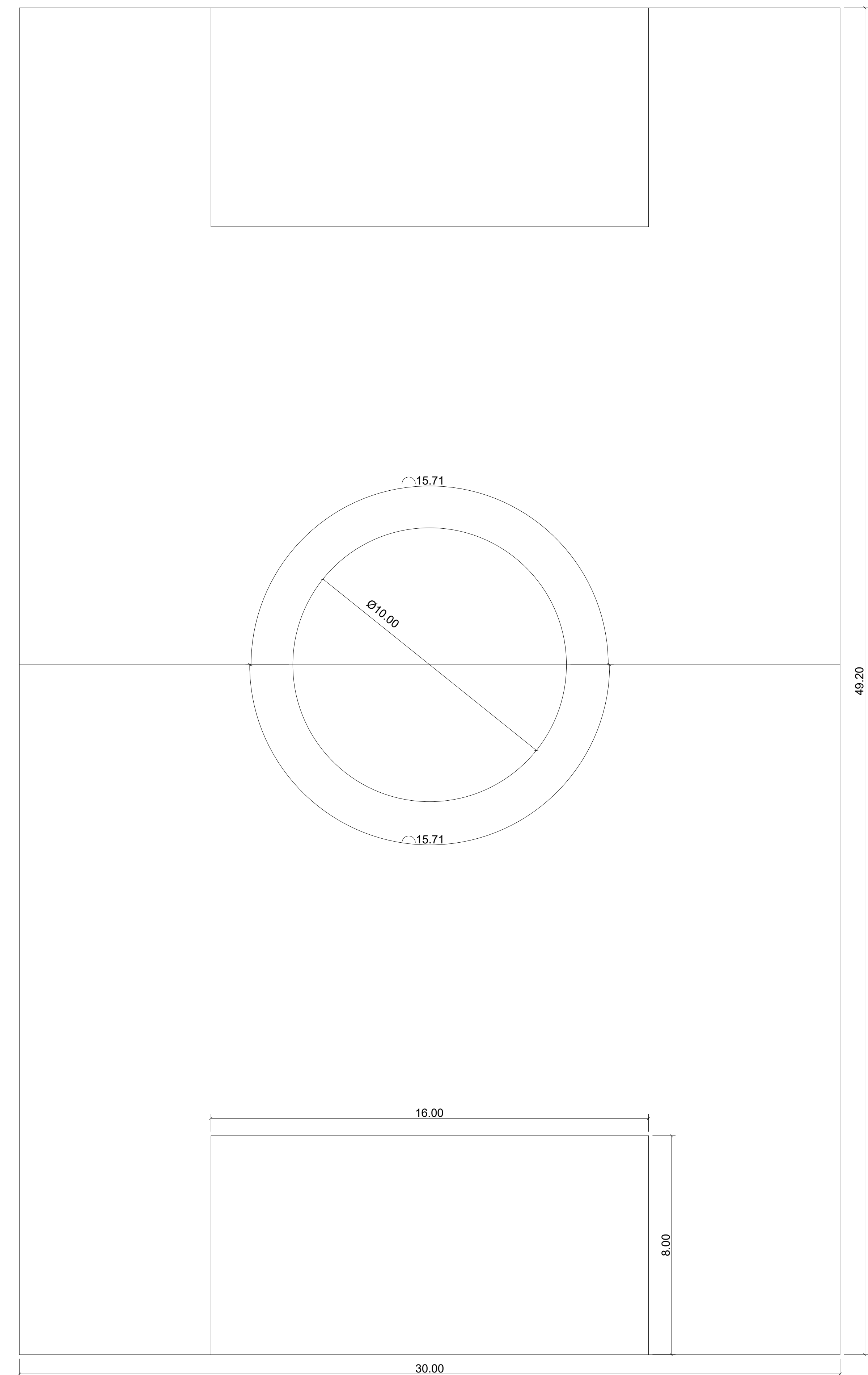
MEDIDAS DAS FAIXAS DEMARCATÓRIAS ESCALA: 1:100
