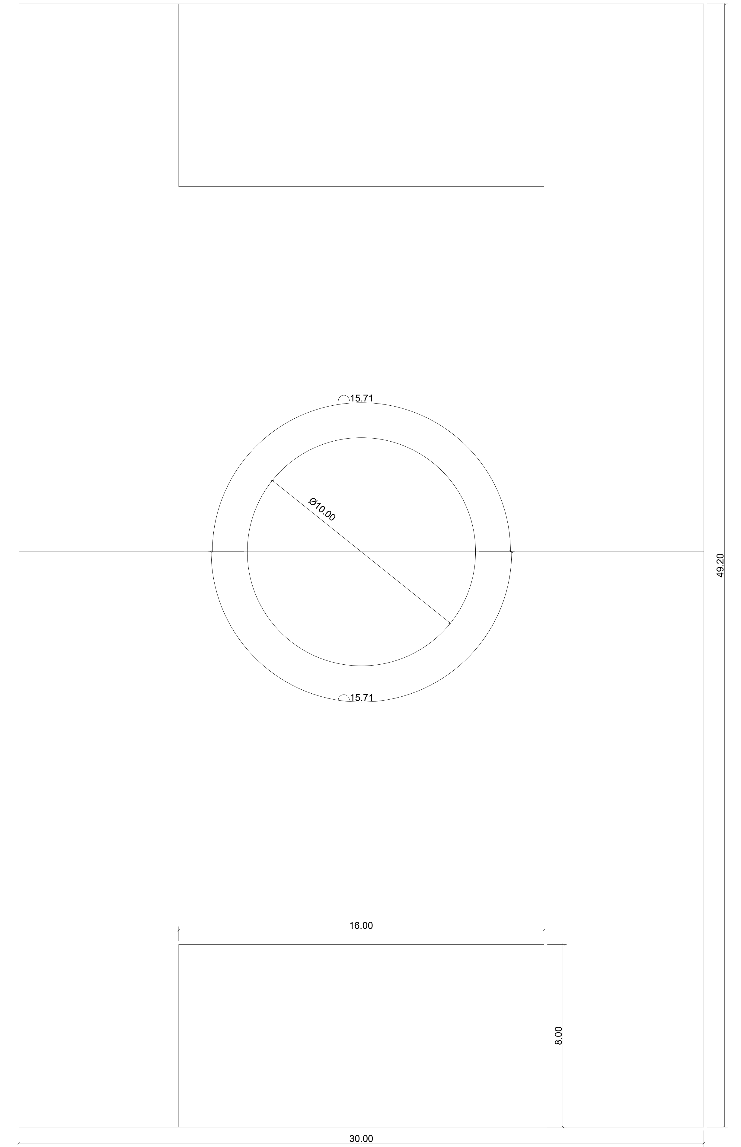
MEDIDAS DAS FAIXAS DEMARCATÓRIAS ESCALA: 1:100
