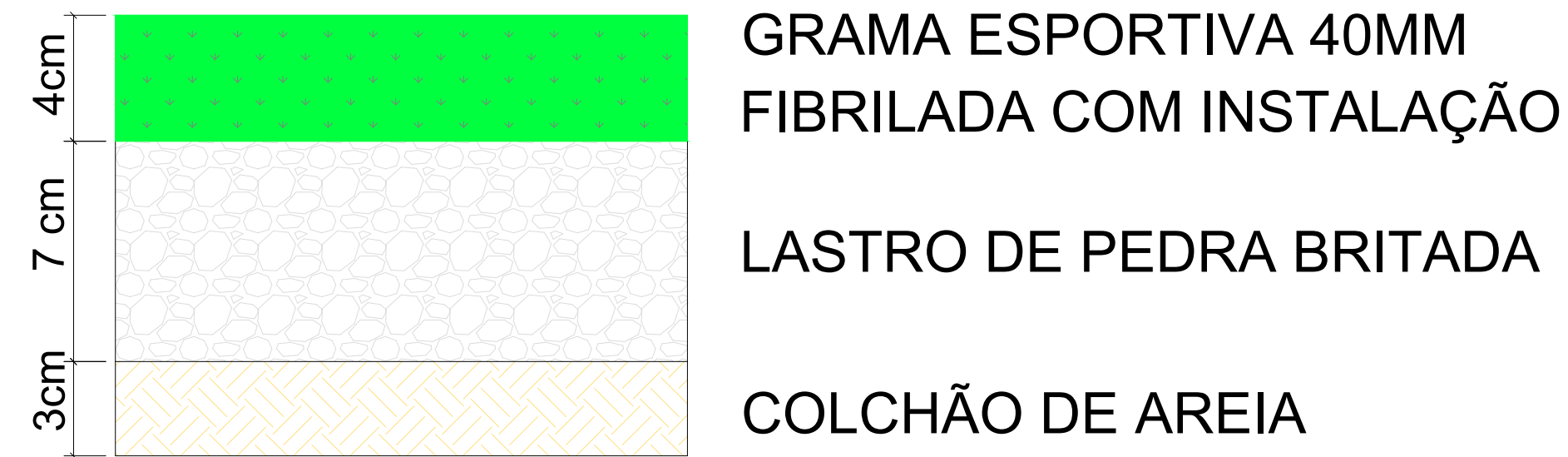
DETALHE INSTALAÇÃO DA GRAMA SINTÉTICA SEM ESCALA
