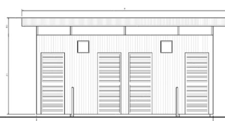
VISTA FRENTE 2 MÓDULOS ACESSÍVEIS / 2 MÓDULOS COMUNS
