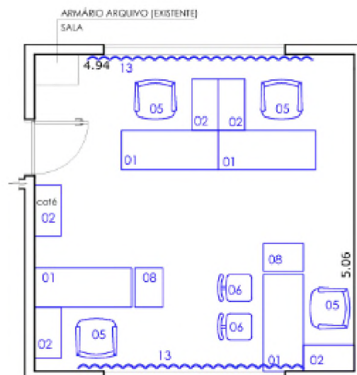
Planta Baixa
