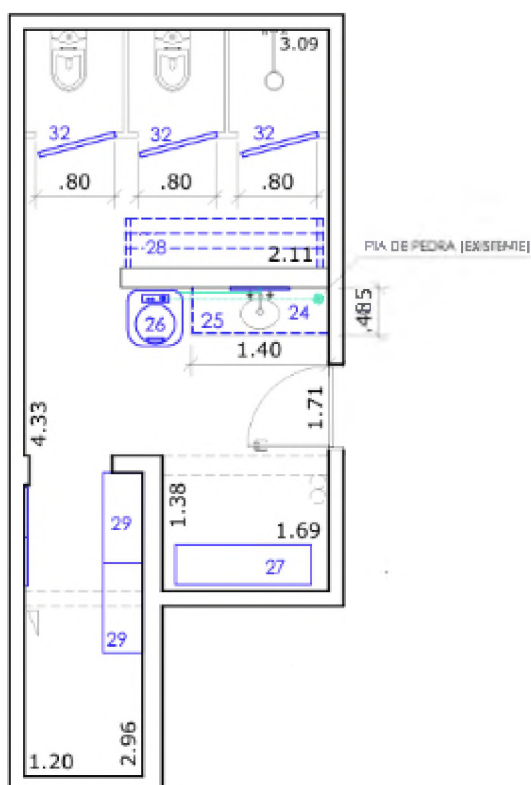
Planta Baixa escala 1:30
