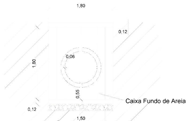
CORTE BB
