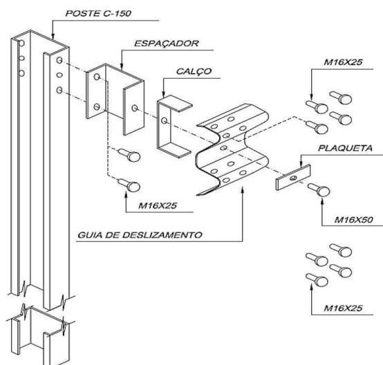
Figura 1 – Componentes da defesa semi-maleável 1
