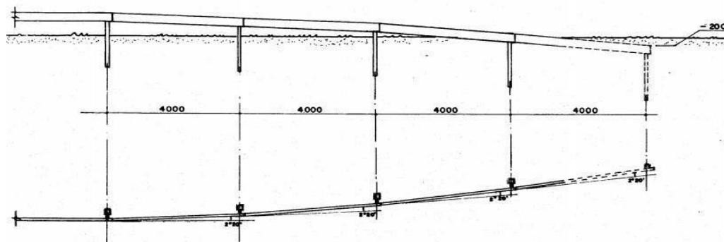
Figura 2 – Ancoragem de defesa
