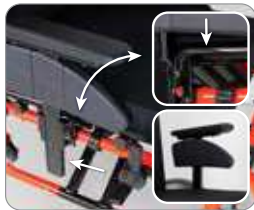
Apoio de braços com ajuste de altura e removível emborrachado. Protetor de roupa de nylon com regulagem de altura e incorporado ao braço.
