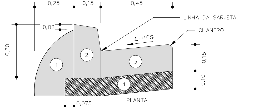
DETALHE DE GUIA E SARJETA 0,45m RECEBENDO SEM ESCALA
