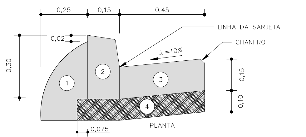
DETALHE DE GUIA E SARJETA 0,45m RECEBENDO SEM ESCALA
