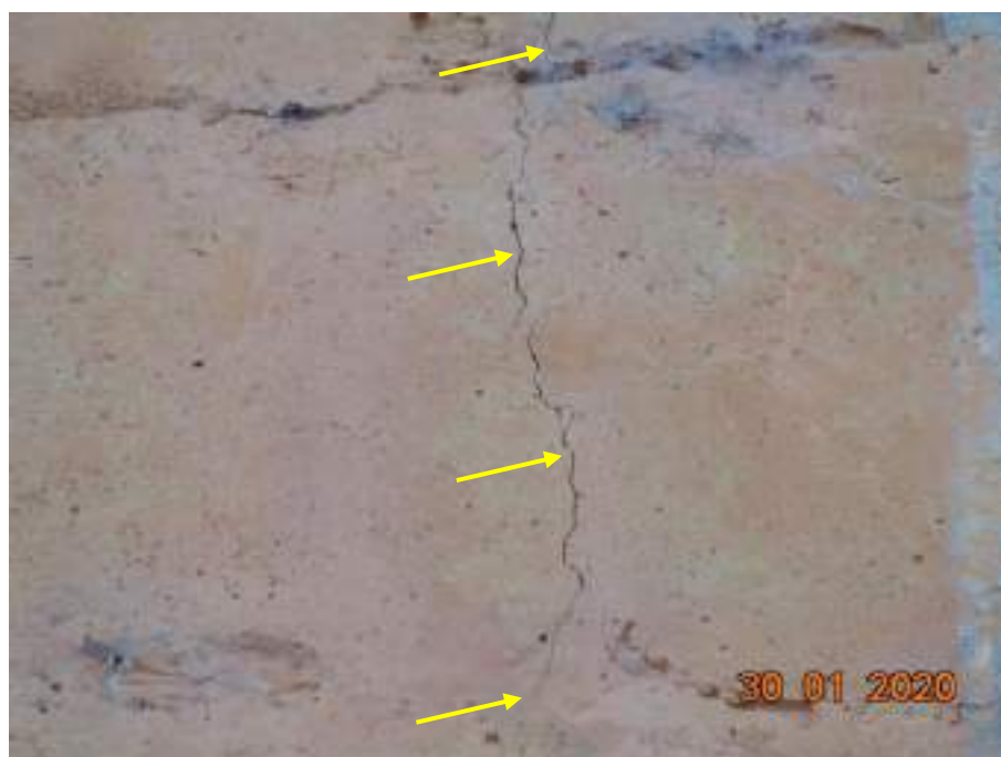
FOTO 188 Fissura com posicionamento vertical e abertura máxima de 0,5mm no pilar P5, face Norte.
