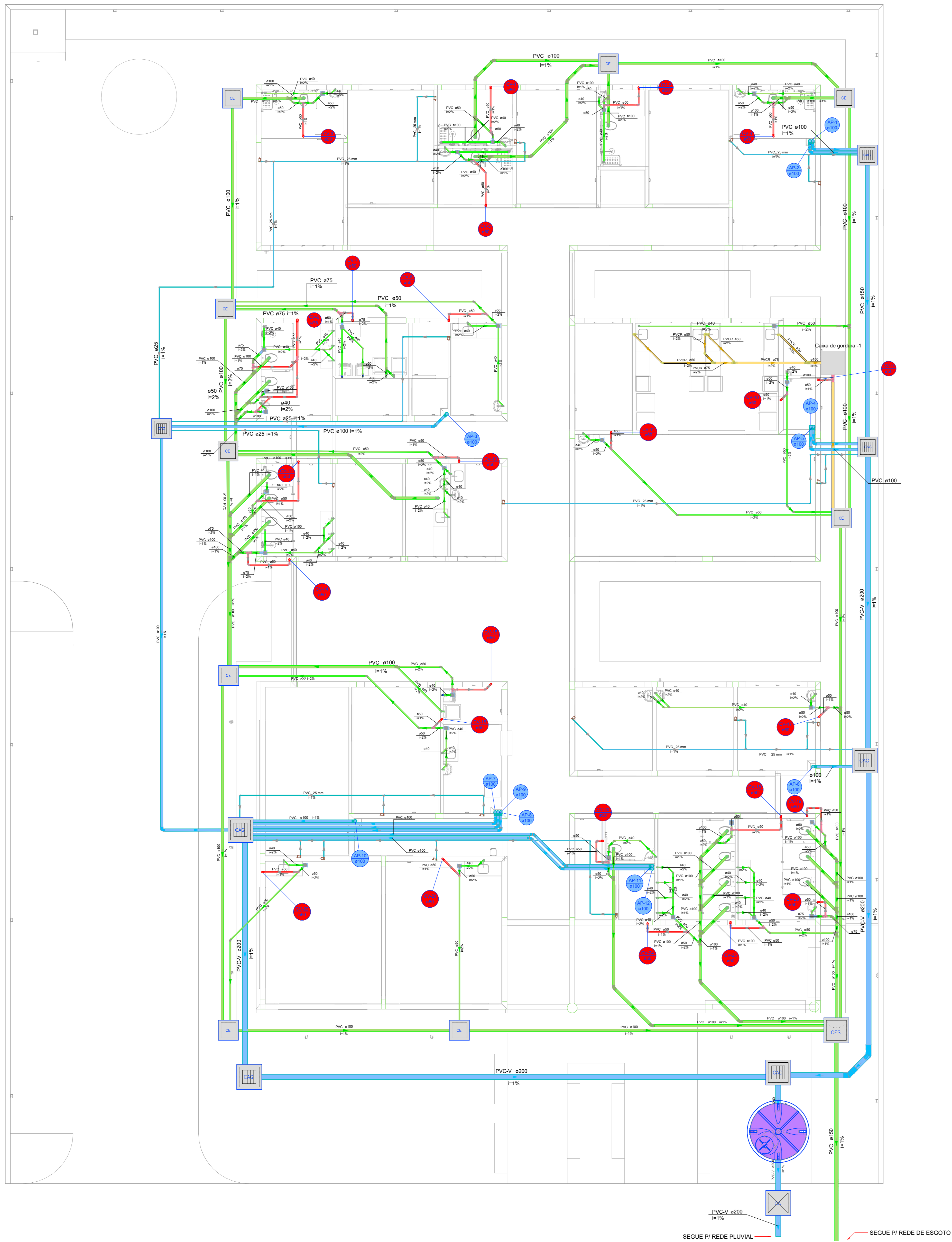
PLANTA - SANITÁRIO - TÉRREO ESC. 1/75
